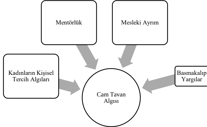
Şekil 1: Çalışmanın Modeli
