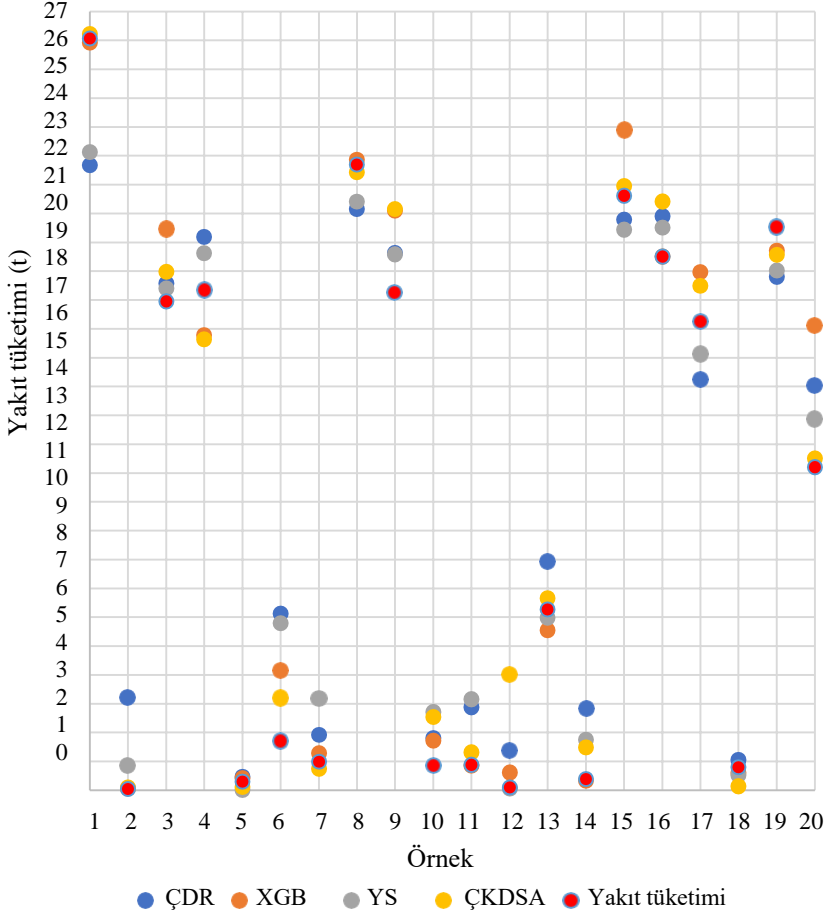
Şekil 6: Rastgele seçilen 20 örnek için yöntemlerin karşılaştırılması
