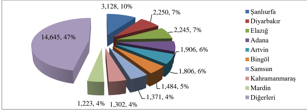
Grafik 16. Türkiye’nin hidroelektrik enerji santrallerine ilişkin bilgiler (MWe) (2022)
