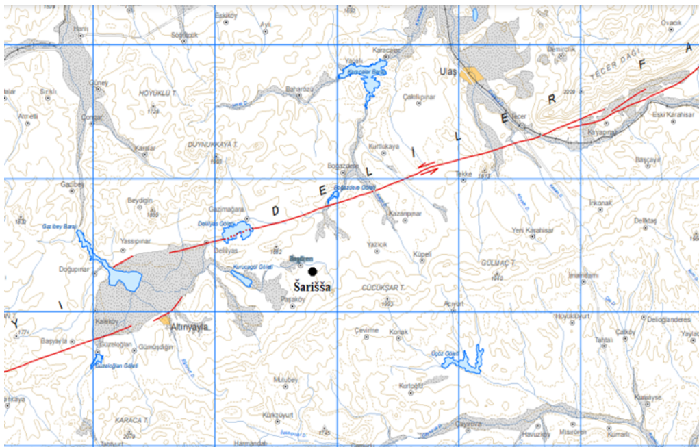
Res. 4: Deliler Fay Hattı ve Şarişsa'nın konumu (MTA Diri Fay Haritaları NJ-37-1 parseli).
