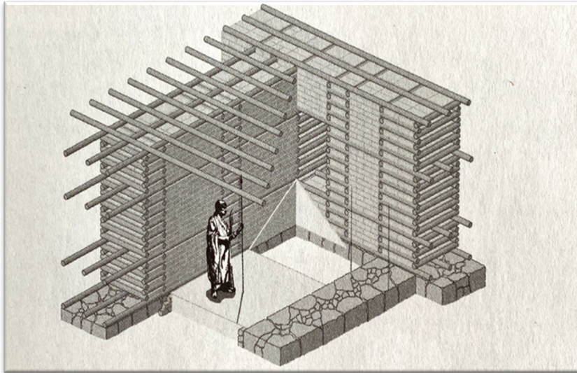
Res. 1: Kamu binalarının inşasında kullanılan ahşap-kil tuğla tekniğı (Mielke, 2019, 97).
