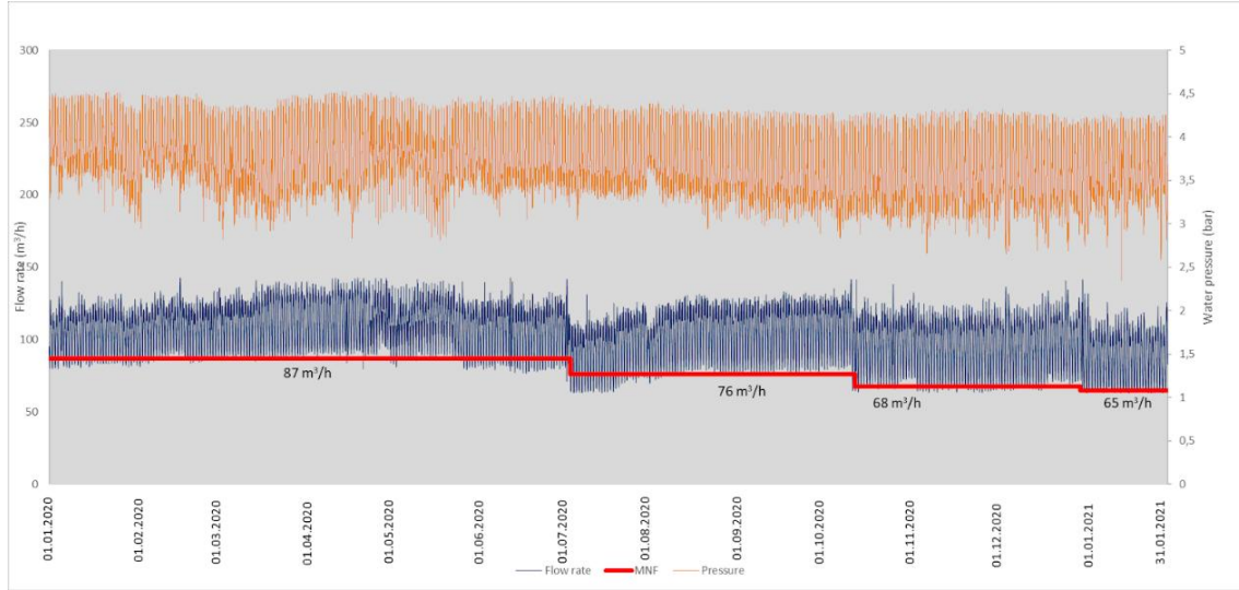
Şekil 2. Çalışma Bölgesi Debi Basınç Değişim Grafiği [3]
