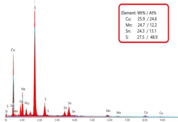
Şekil 6. CMTS ince filminin EDX analizi ile Elementel kompozisyonu
