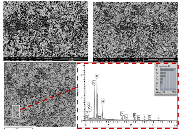
Şekil 5. D(x=0.15) örneğinin farklı büyütmelerdeki (soldan sağa doğru 5000x ve 2500x ) yüzey SEM görüntüleri. Alttaki satır ise D-örneğinin EDX analiz sonucu.
