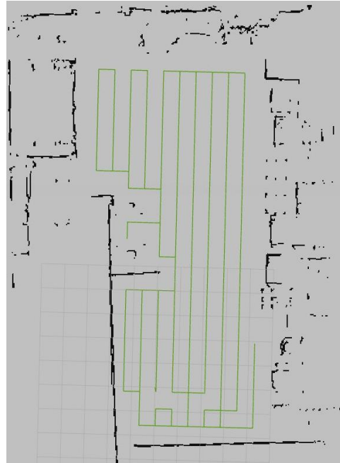
Şekil 2. Klasik Boustrophedon Yol Planı
