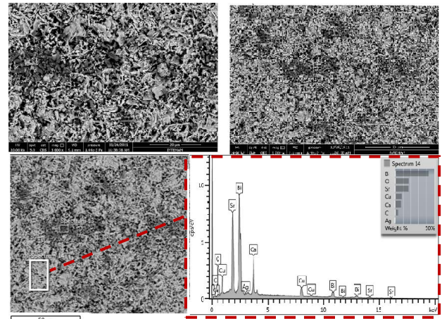
Şekil 6. E (x=0.20) örneğinin farklı büyütmelerdeki (Soldan sağa doğru 5000x ve 2500x) yüzey SEM görüntüleri. Alttaki satır ise E-örneğinin EDX analiz sonucu.
