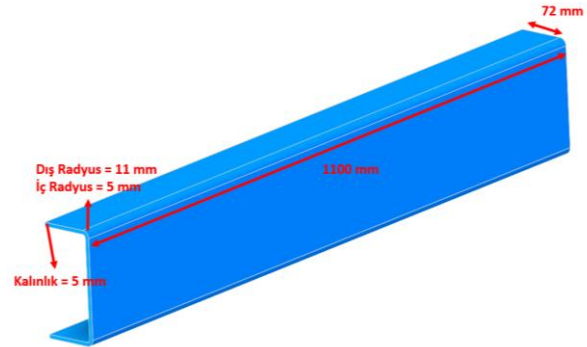
Şekil 3. Araç şasisinde kullanılan orta kısımdaki C profil ölçüleri
