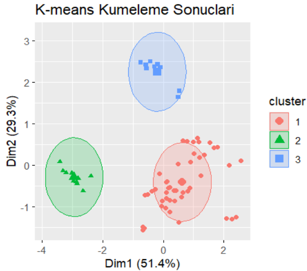
Şekil 5. Kümeleme Sonucunun Görselleştirilmesi
