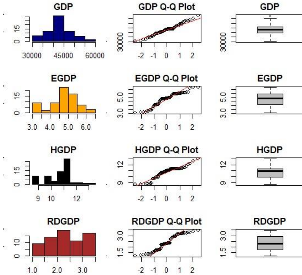
Şekil 2. Değişkenlere Ait Histogram, QQ Plot, Kutu Grafikleri
