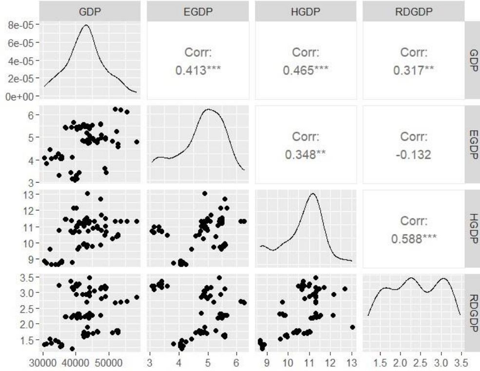
Şekil 3. Pairwise Korelasyon Matrisi Ve Dağılım Grafikleri
