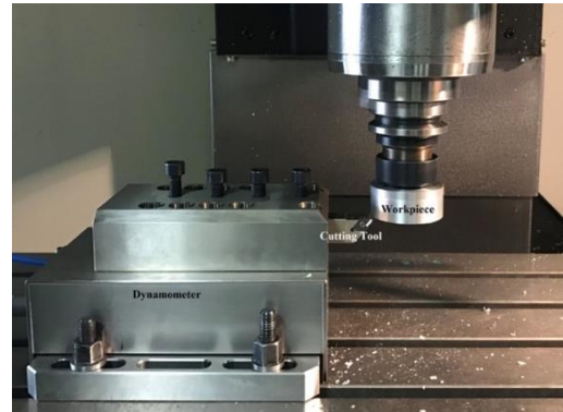
Şekil 1. Deney düzeneği
