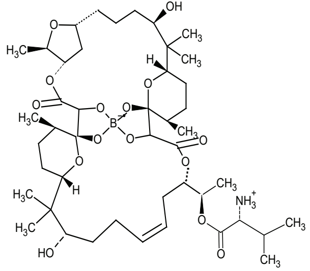
Şekil 2. Boromisin bileşiğinin yapısı (Structure of boromycin compound).
