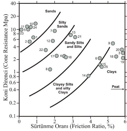
Şekil 8. İncelenen örneklerin Robertson ve Campanella [16] sınıflama abağı içerisindeki dağılımları
