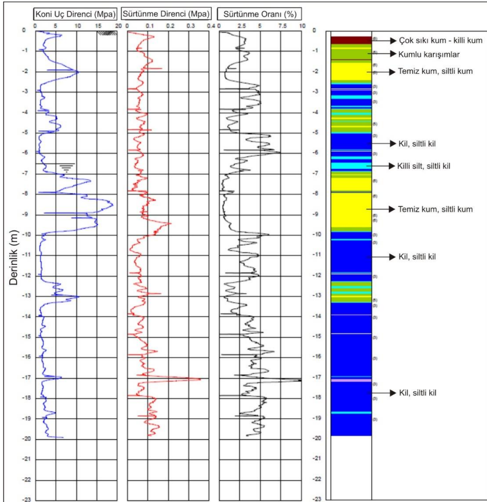
Şekil 4. CPT-1 ölçüm lokasyonu örneğinde elde edilmiş deney verileri ve olası zemin profili
