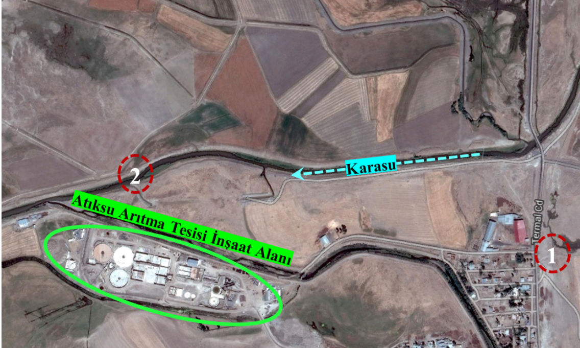
Şekil 6. Ilıca kollektör (1) ve ham atıksu deşarj noktasında (2) Karasu nehrinin numunelerinin alındığı noktalar.
