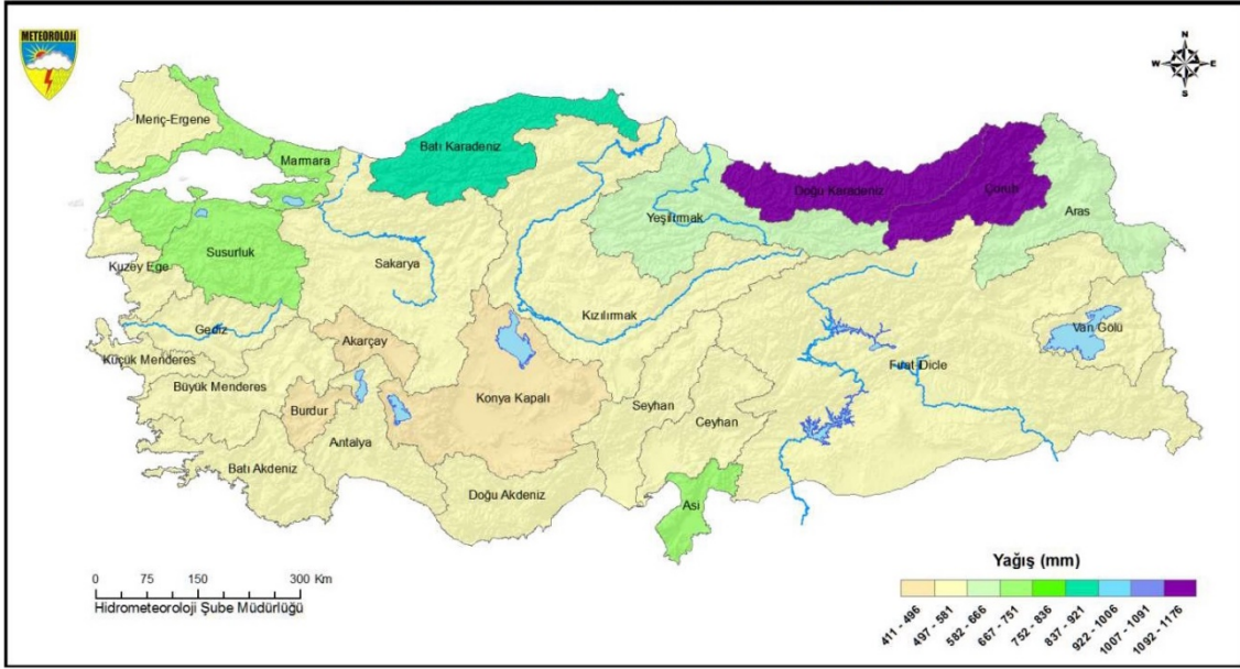
Şekil 2. Havza bazlı yağış haritası.
