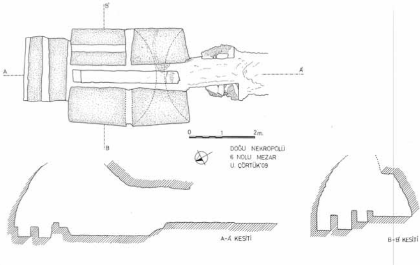
Levha 2. 6 no.lu kaya mezarının çizimi.
