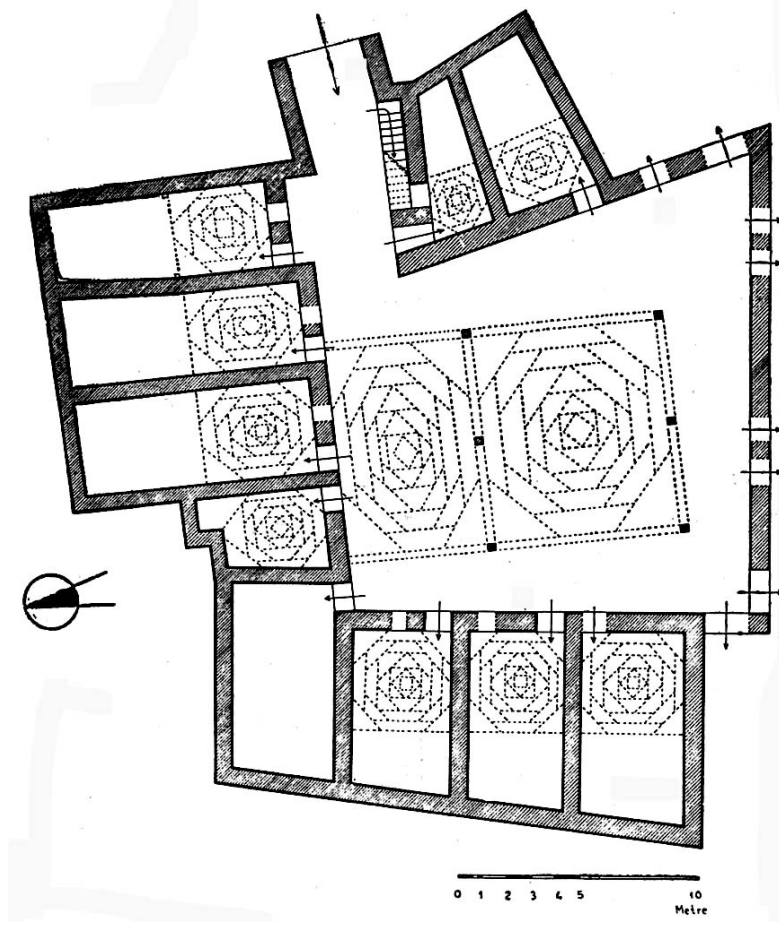
Çizim1: Cennetzade Hanı (R. H. Ünal'dan)
