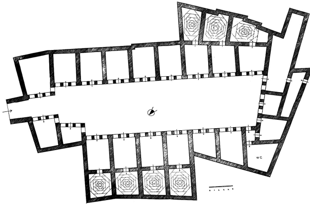
Çizim 6: Kamburoğlu Hanı (R. H. Ünal'dan)
