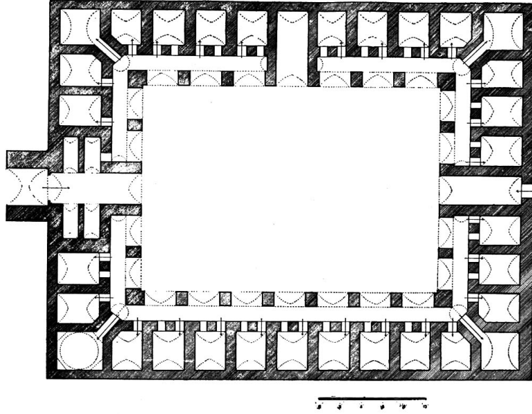
Çizim 7: Rüstem Paşa Kervansarayı Zemin Kat (R. H. Ünal'dan)
