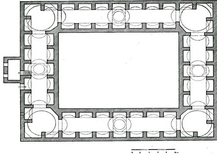
Çizim 8: Rüstem Paşa Kervansarayı Birinci Kat (R. H. Ünal'dan)
