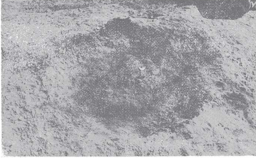
Res. 3 — Tepe III, Geç Demir Çağı Açık Hava Çömlekçi Fırını
