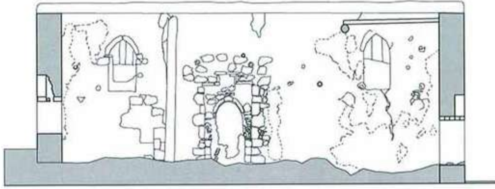
Şek. 8. Çullu köyü camisi (env. no: K16.C5.1), enine kesit, rölöve.
