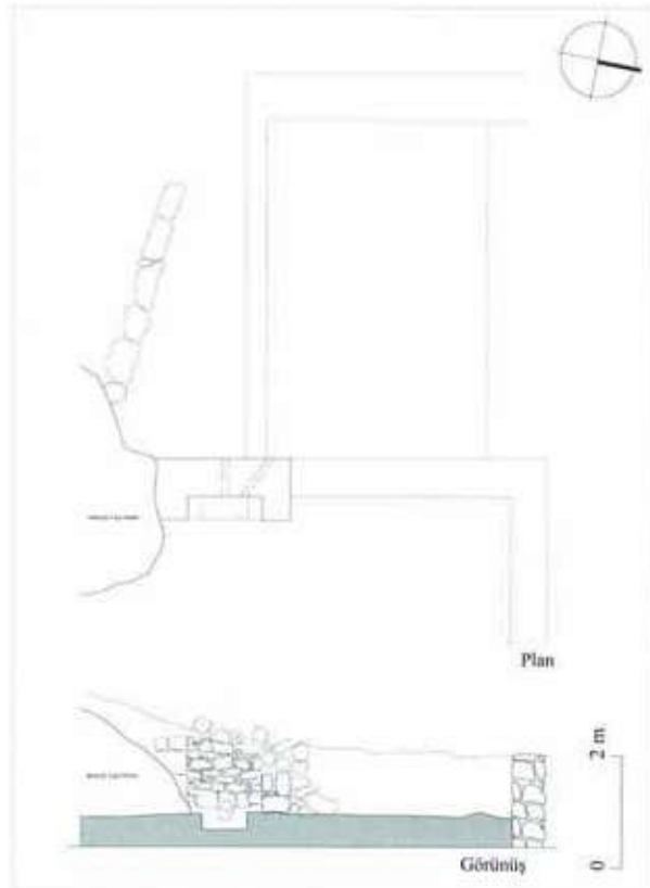
Şek. 13. Çullu köyü, çeşmecik (env. no: K16.C5.5) ve havuzu (env. no: K16.C5.6), rölöve planı.
