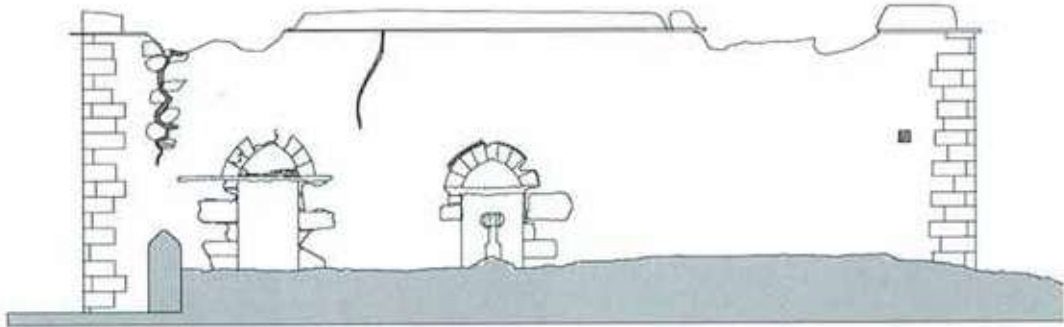
Şek. 10. Çullu köyü camisi, doğu cephesi, rölöve.
