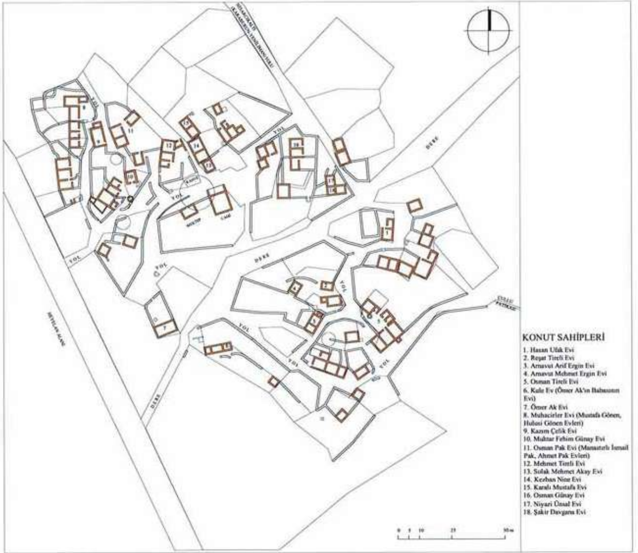
Şek. 3. Hisarcık köyü yerleşim planı, ön-restitüsyon. Plan için kadastral harita esas alınmıştır.
