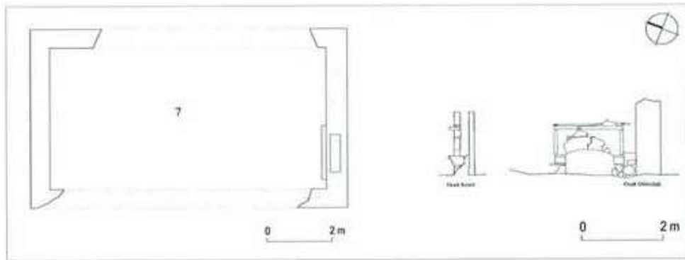
Şek. 11. Hisarcık köyü, Ömer Ak Evi (env. no: K16.C5.62), rölöve.
