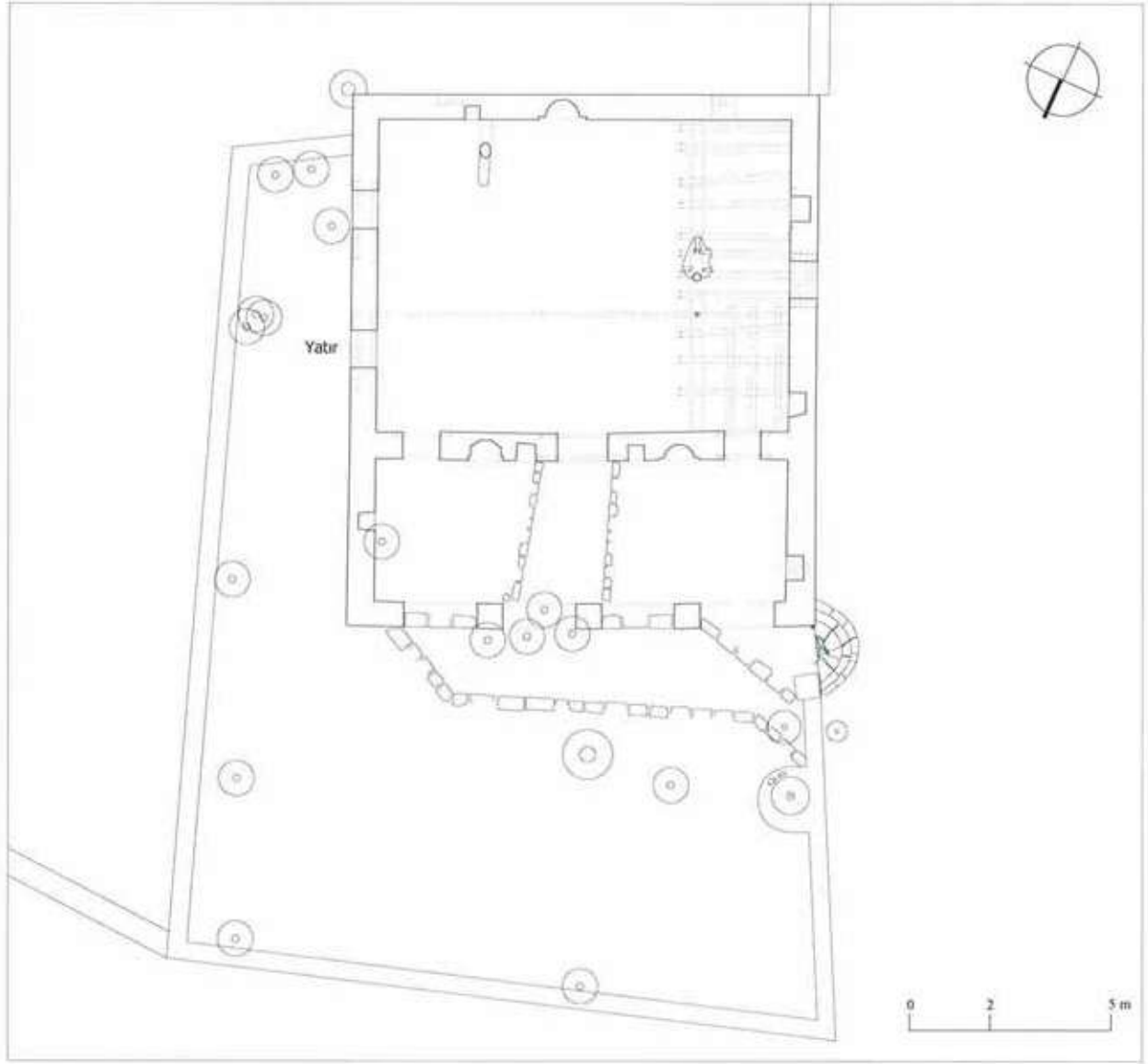
Şek. 6. Çullu köyü camisi (env. no: K16.C5.1), rölöve planı.
