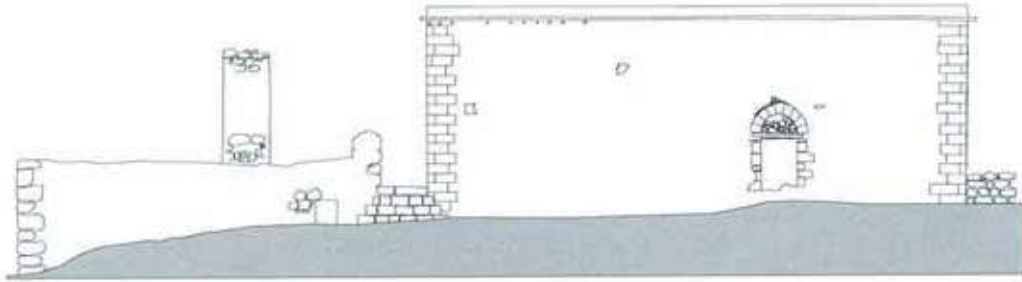
Şek. 9. Çullu köyü camisi, batı cephesi, rölöve.
