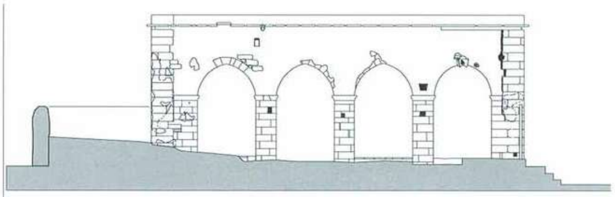
Şek. 7. Çullu köyü camisi, revak cephesi, rölöve.
