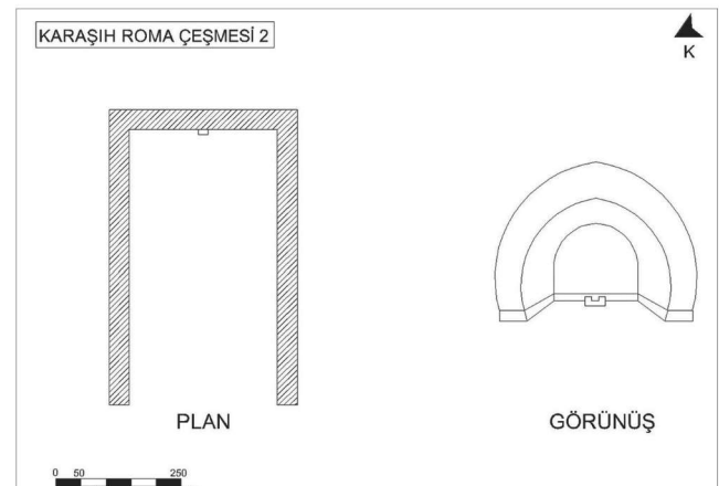
Şekil 10 - Sumbas, Karaşih Roma Çeşmesi 2 Çizim / Sumbas, Karaşih Roman Fountain 2 drawing
