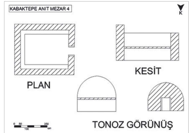
Şekil 8 - Sumbas, Kabaktepe Anıt Mezar 4 / Sumbas, Kabaktepe Monumental Grave 4
