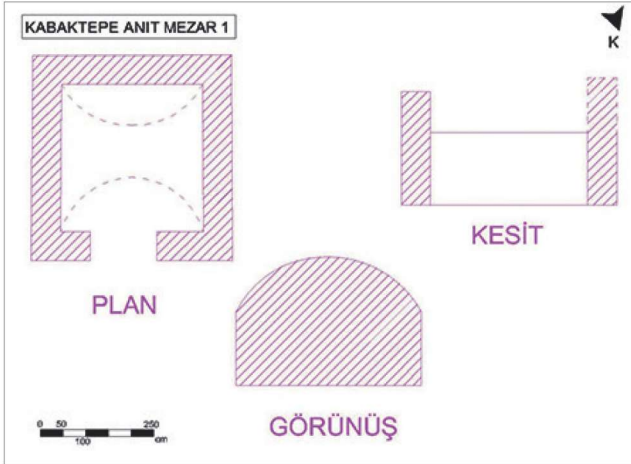
Şekil 4 - Sumbas, Kabaktepe Anıt Mezar 1 / Sumbas, Kabaktepe Monumental Grave 1
