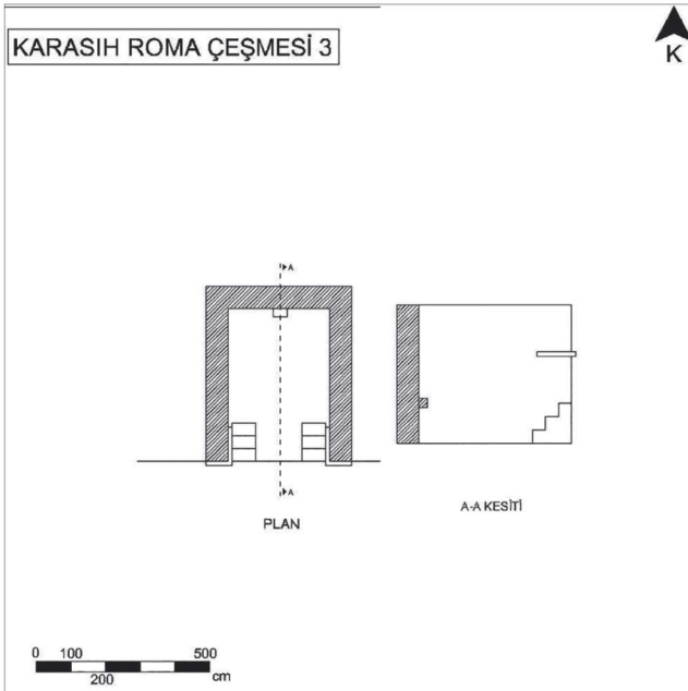
Şekil 11 - Sumbas, Karashih Roma Çeşmesi 3 Plan / Sumbas, Karashih Roman Fountain 3 plan
