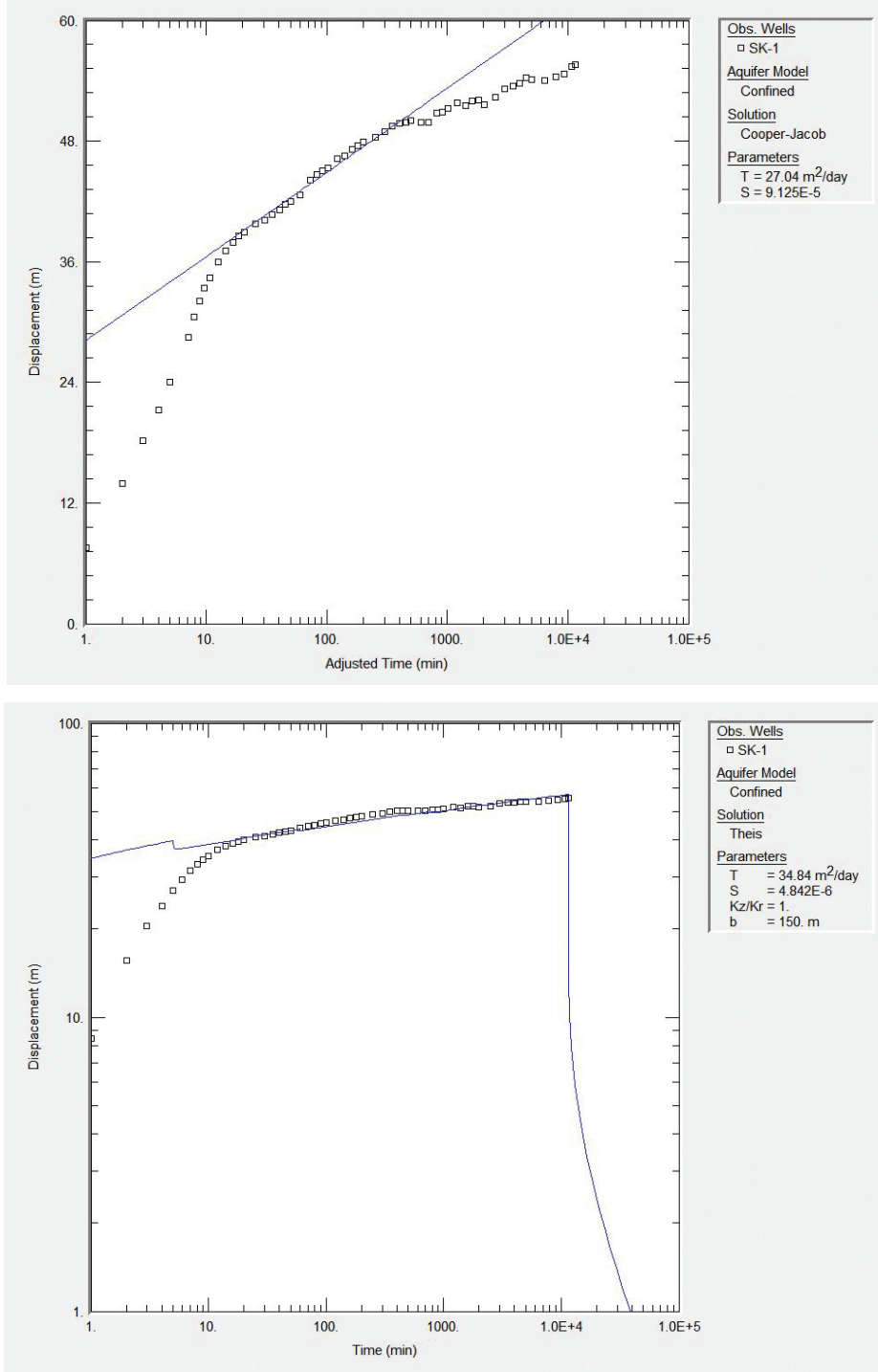
Şekil 6. Sayısal çözüm sonuçları (Cooper and Jacob, 1946 ve Theis). Figure 6. Numerical solution results (Cooper and Jacob, 1946 and Theis).
