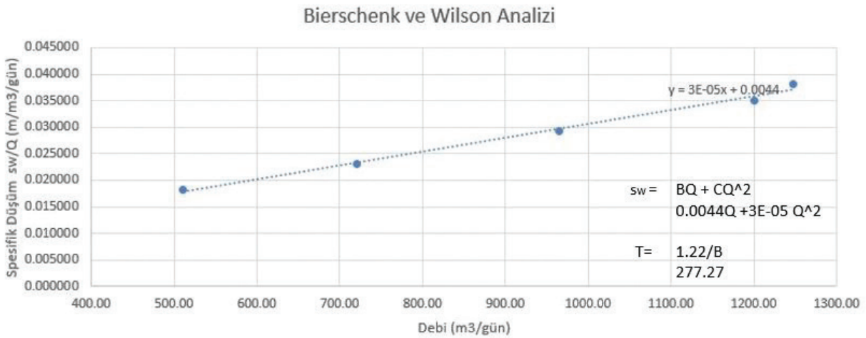
Şekil 3. Biershenk ve Wilson analizi.
