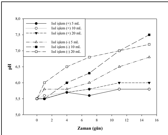
Şekil 5. Tüm reaktörlerde pH değişimleri.
