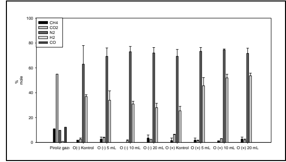
Şekil 6. Reaktörlerde tep gazı kompozisyonları (O(-): Isıl ön işlemsiz; O(+): Isıl ön işlemlili).
