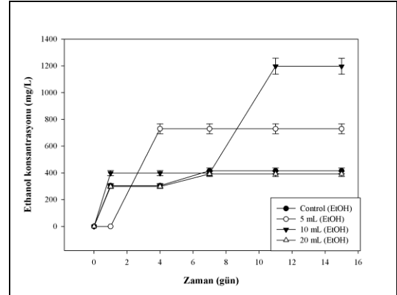
Şekil 3. Isıl ön işlemsiz karışık kültür ile etanol üretimi.
