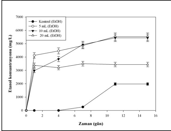
Şekil 1. Isıl ön işlem uygulanmış karışık kültür ile etanol üretimi.
