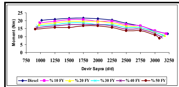
Şekil 4. Diesel yakıtı ve fındık yağı / Diesel yakıtı karışımlarının motor devir sayısına bağlı olarak moment değerlerinin değişimi
