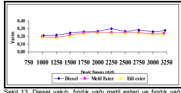
Şekil 13. Diesel yakıtı, fındık yağı metil esteri ve fındık yağı etil esteri yakıtlarının motor devir sayısına bağlı olarak toplam verim değerlerinin değişimleri
