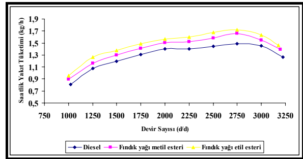
Şekil 9. Diesel yakıtı, fındık yağı metil esteri ve fındık yağı etil esteri yakıtlarının motor devir sayılarına bağlı olarak saatlik yakıt tüketimlerinin değişimleri
