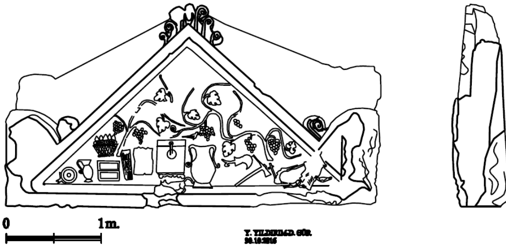
Çizim 4. Safranbolu Kalesi, Roma Dönemi Mezar Anıtı (Yıldırım ve Gür, 2016)
