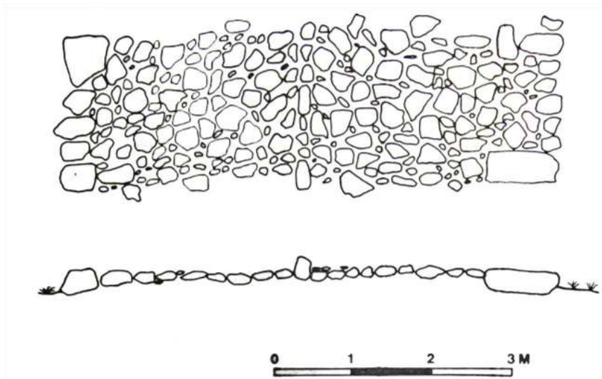
Çizim 6. Düz Bir Alanda İnşa Edilen Yol Plan ve Kesiti (French, 1981: 23, Şekil 1)
