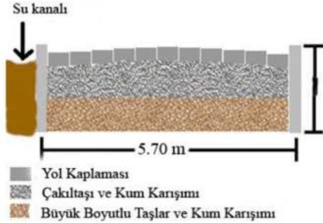
Çizim 5. Roma Yol Kesiti (Pehlivan, 2010: Levha I-Çizim 1)
