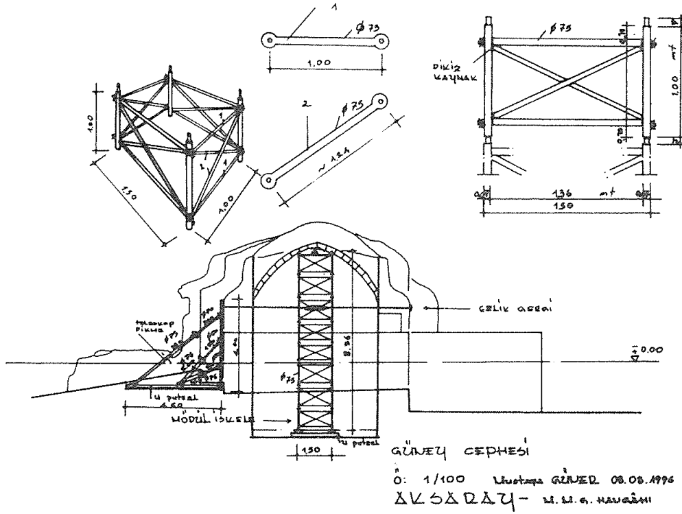
Şek. 17- Aksaray-Melik Mahmud Gazi Hangârı, destekleme projesi, 1996.
