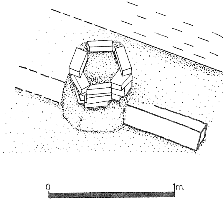
Şek. 14- Aksaray-Melik Mahmud Gazi Hangâhı, kuzey yönü, ana beden duvarı üzerine yapılmış tuğla ocak, XVIII-XIX. yy., 1996.
