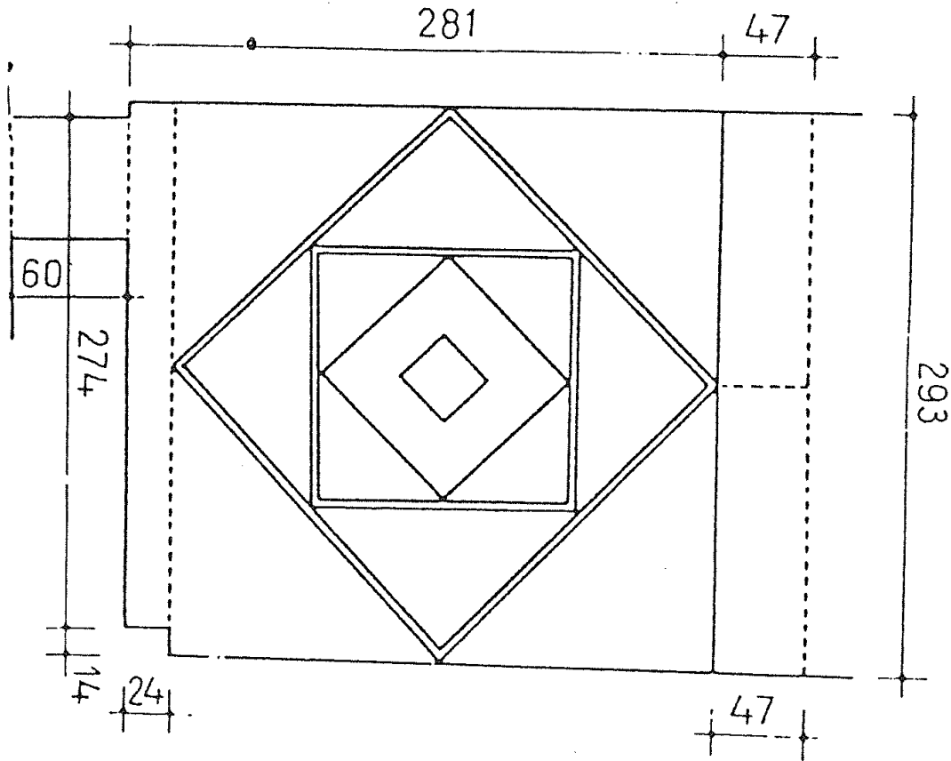
Şek. 3- Aksaray-Melik Mahmud Gazi Hangâhı, giriş eyvanı üstündeki ikinci katın ikinci odasının üst örtüsü (A. Tükel Yavuz'dan).
