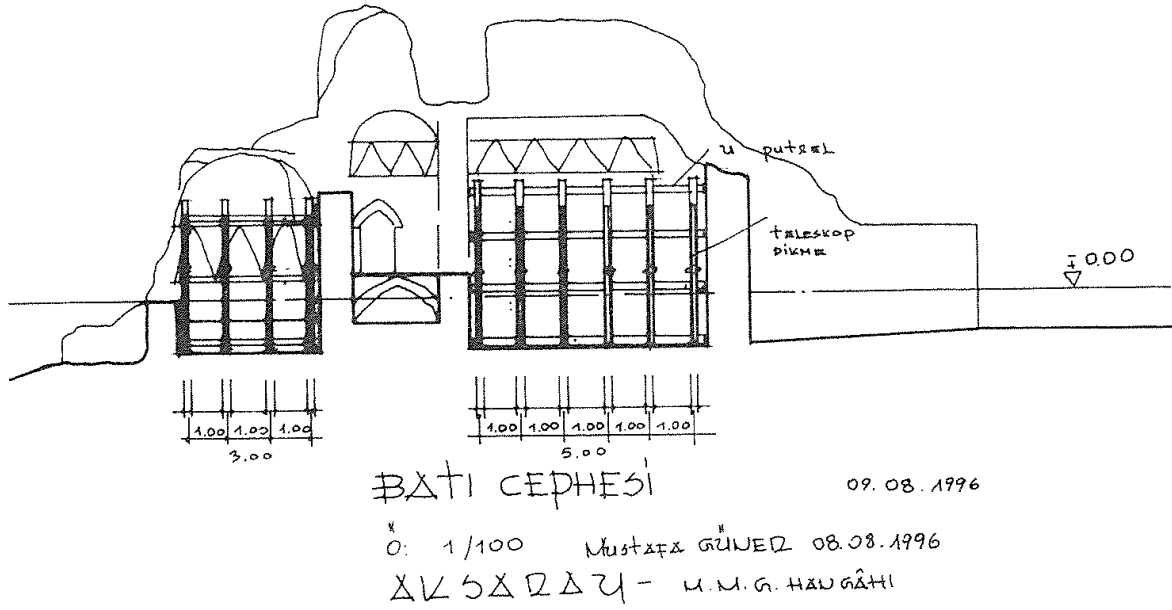
Şek. 18- Aksaray-Melik Mahmud Gazi Hangâhı, destekleme projesi, 1996.
