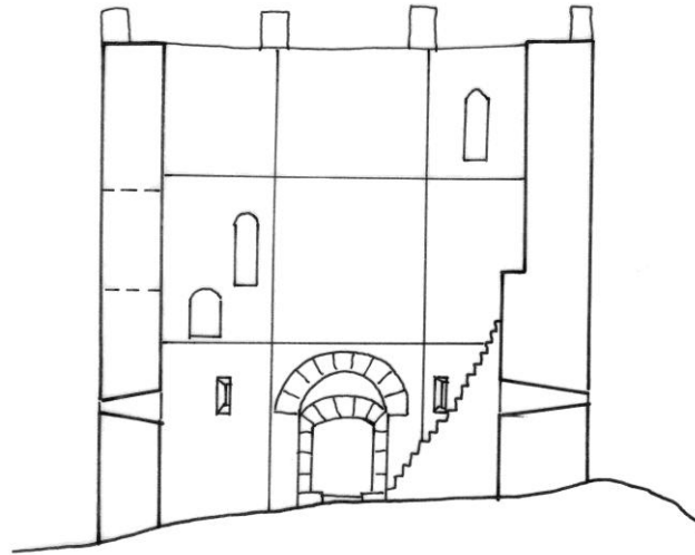
D-D kesiti
