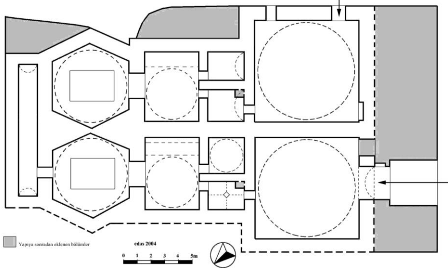
Şek. 1- Menemen, Karakadı (Altı Kardeşler) Hamamı. Plan.
