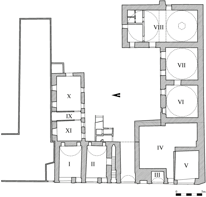
Şekil 1- Gölarmara Halime Hatun İmaret. Zemin kat rölövesi (Y. Mim. U. D. Genç'ten işlenerek)
