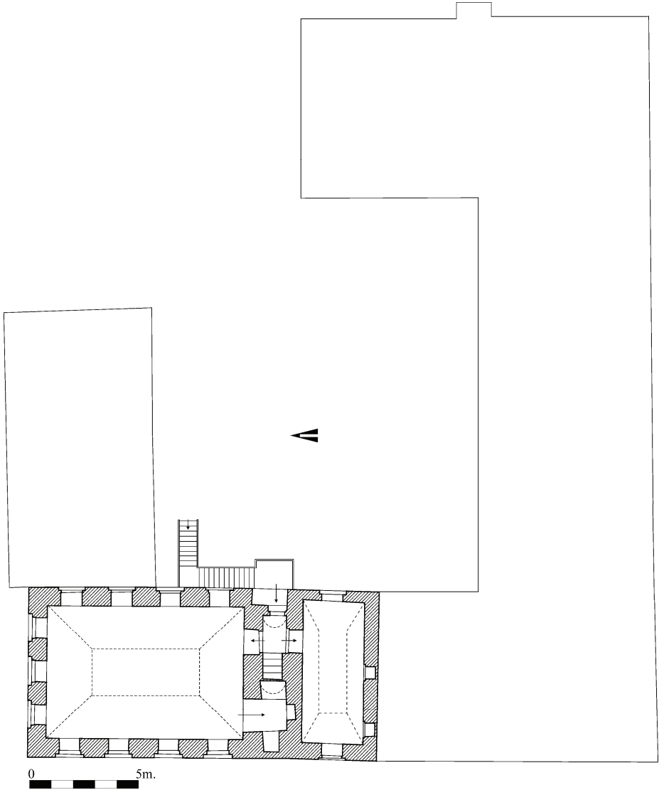
Şekil 4- Gölarmara Halime Hatun İmaretı. Birinci kat restitüsyon önerisi. (Y. Mim. U. D. Genç'ten işlenerek).
