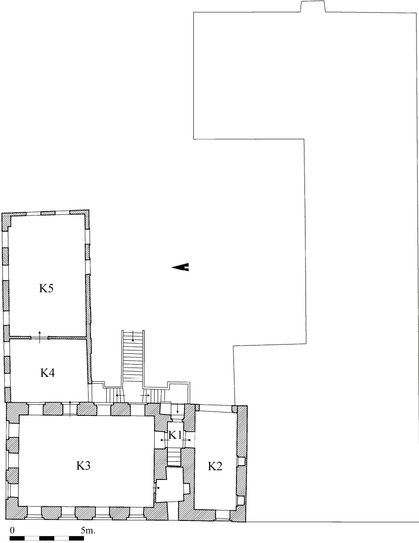
Şekıl 2- Gölmarmara Halıme Hatun İmaretı. Bırınçı kat rölövesı (Y. Mım. U. D. Genç'ten işlenerek)
