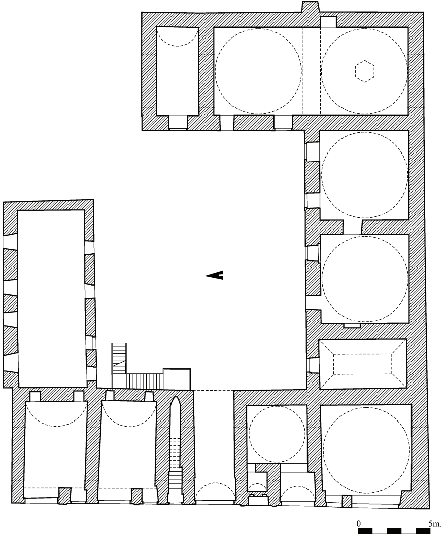
Şekil 3- Gölmarmara Halime Hatun İmareti. Zemin kat restitüsyon önerisi. (Y. Mim. U. D. Genç'ten işlenerek).
