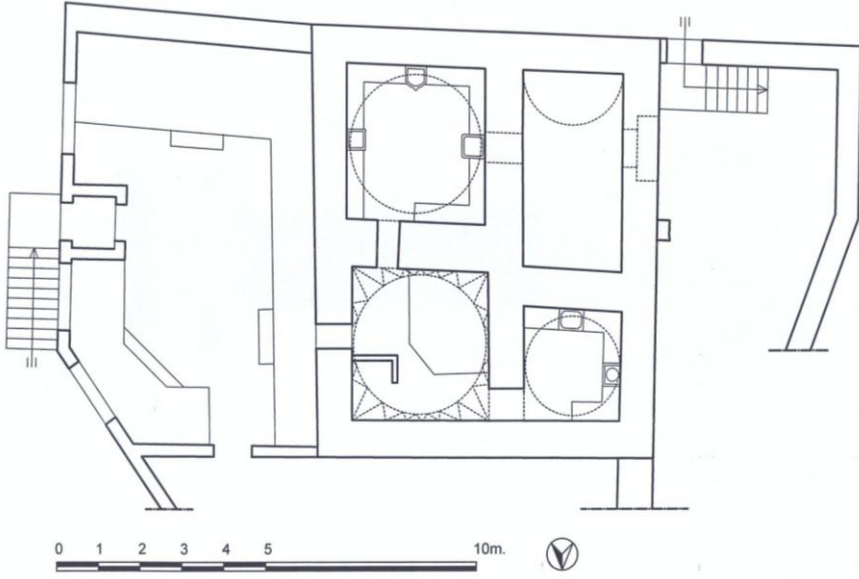
Şek.2- Metrük hamamın planı
