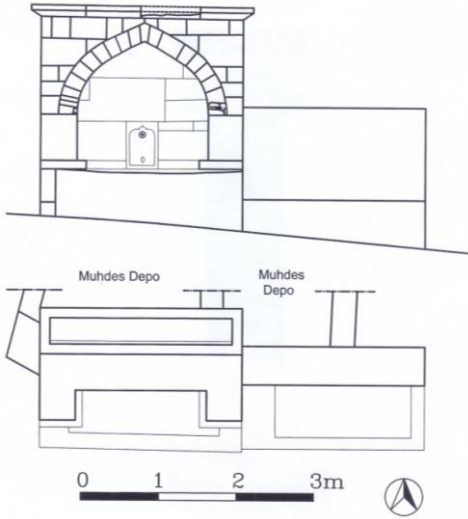
Şek.4- Kadı Çeşmesi, plan ve cephe.
