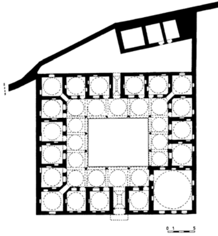
Şek.1- Damat İbrahim Paşa Medresesi planı (İ. Aktuğ'dan).
