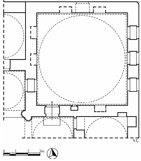
Şek.2-Damat İbrahim Paşa Medresesi Kütüphanesi planı.
