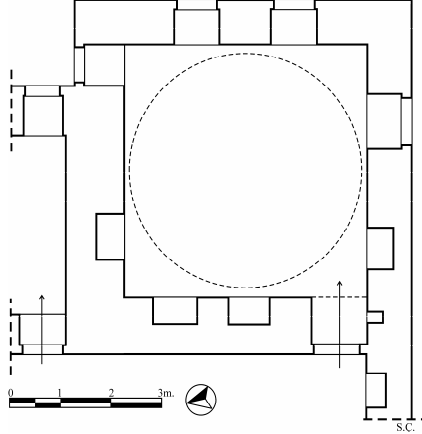
Şek.4- Karavezir Seyyid Mehmet Paşa Medresesi Kütüphanesi planı.
