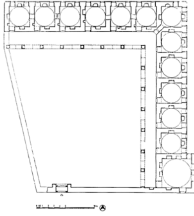
Şek.3- Karavezir Seyyid Mehmet Paşa Medresesi planı (M. Sözen-vd.'nden).
