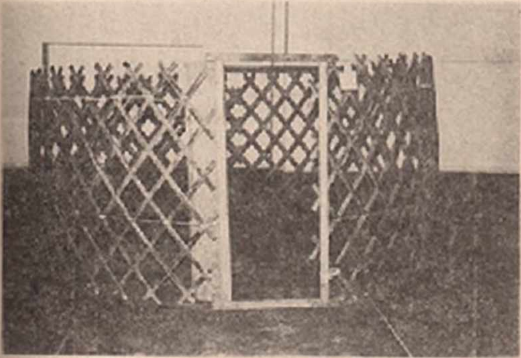
Fotoğraf 4. Kanatların, çadırın yan yüzünü oluşturacak şekilde kurulmuş görünümü.
