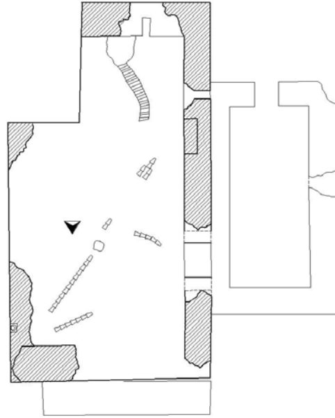
Şekil 6: Antalya-Burdur Evdir Han Planı (O.Eravşar'dan)
