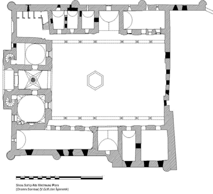
Şekil 2: Sivas Sahip Ata (Gök) Medresesi Planı.
