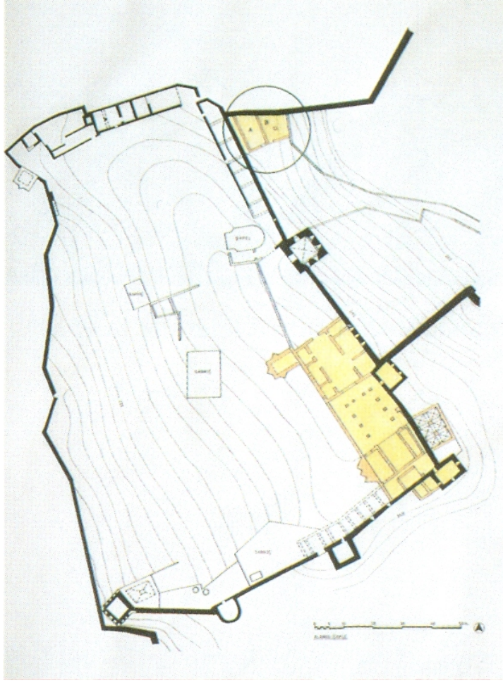
Şekil 12: Alanya Selçuklu Sarayı Planı (M.O.Arık'tan).
