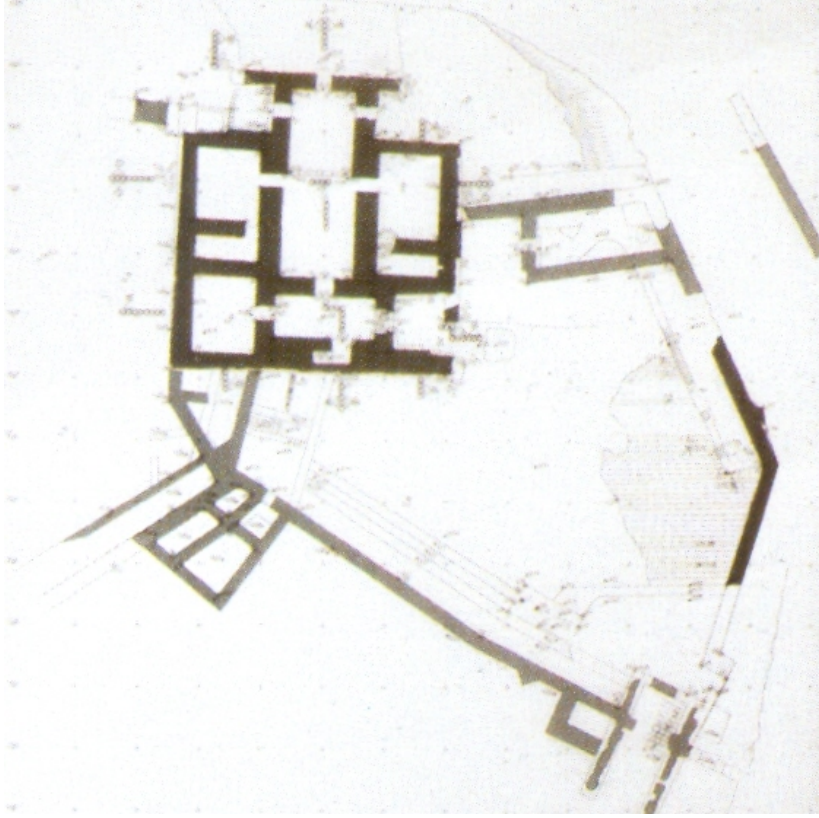
Şekil 10: Kubad-Abad Büyük Saray Planı (Otto-Dorn'dan).
