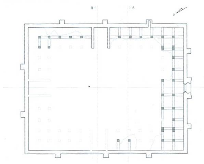
Şekil 6: Antalya-Burdur Evdir Han Planı (O.Eravşar'dan)
