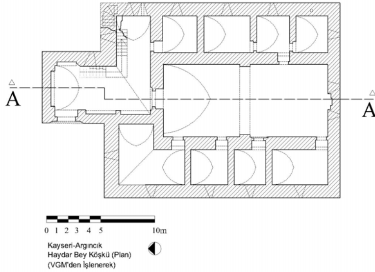
Şekil 8: Kayseri Haydar Bey Köşkü Planı.
