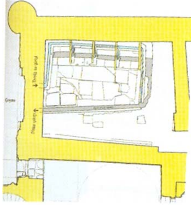
Şekil 3: Sivas Sahip Ata (Gök) Medresesi tuvalet mekânı planı (Y.Kahya'dan).
