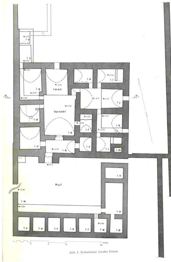
Şekil 11: Isparta Yenişarbademli Malanda Köşkü Planı.
