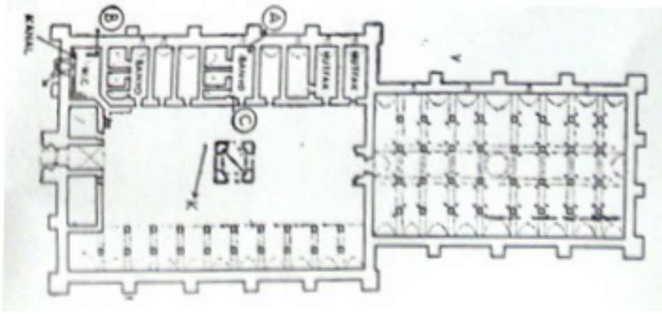
Şekil 5: Aksaray Sultan Hanı Planı (O.C.Tuncer'den).
