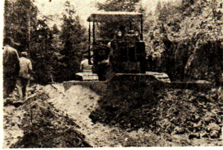
ŞEKİL 13. Karadere (Bolu) orman yolunda International TD 14 tipi Dozerle (kablo kontrollü) inşaat
