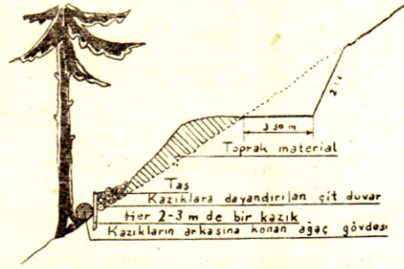
ŞEKİL 1. Dereye yolun aşağısında kalan ormanın yuvarlanan taşlara karşı korunması
