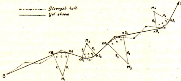
ŞEKİL 5. Kavis baş ve ara noktalarının bulunmasıyla yol ekseninin elde edilmesi
