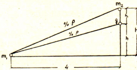
ŞEKİL 3. İki esas nokta arasında tatbik edilmesi lâzım gelen meyil nisbetinin bulunması
