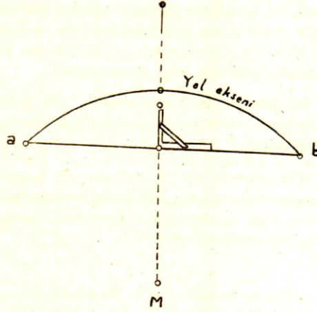
ŞEKİL 8. Kavislerde profil noktalarında en kesit istikametinin belli edilmesi
