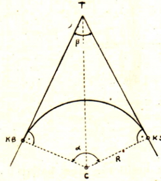
ŞEKİL 4 b. Merkez açısının bulunması
