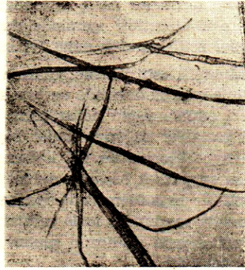
ŞEKİL 3. Çam odunundan yarı kimyevi selüloz metoduna göre elde edilmiş olan selüloz lifleri
