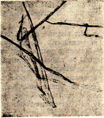
ŞEKİL 2. Lâdin odunundan sülfat metoduna göre elde edilmiş olan selüloz lifleri
