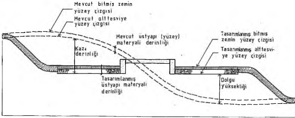
Resim 4.1: Mevcut ve tasarlanmış üst yüzey materyali ile kazı ve dolgu hacimleri arasındaki ilişki
