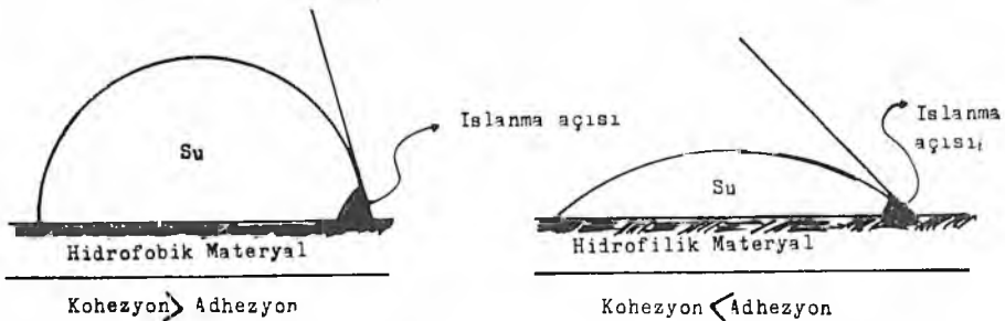
Şekil 3. Hidrofobik ve Hidrofilik Materyaller Üzerinde İslanma Açılarının Şematik Gösterilmesi.
