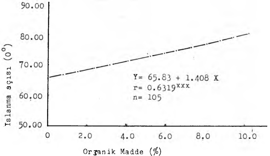
Şekil 5. Metamorfik Şist Anamateryalden Gelişmiş Topraklarda Organik Madde ile Islanma Açısı Arasındaki İlişki (ŞENGÖNÜL 1984).
