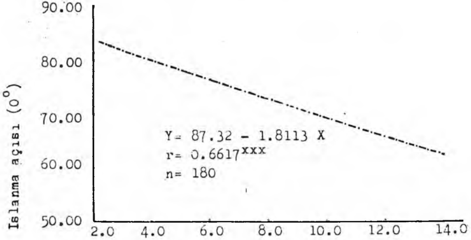
Şekil 6. Granit Anamateryalden Gelişmiş Topraklarda Kıl Miktarı İle İslanma Açısı Arasındaki İlişki (ŞENGÖNÜL 1984).
