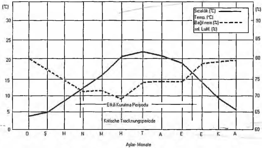
Şekil 7: Düzcce'de 10 yıllık (1978-1988) sıcaklık ve bağılnem ortalamalarına göre çizilen etkili kurutma periyodu.
