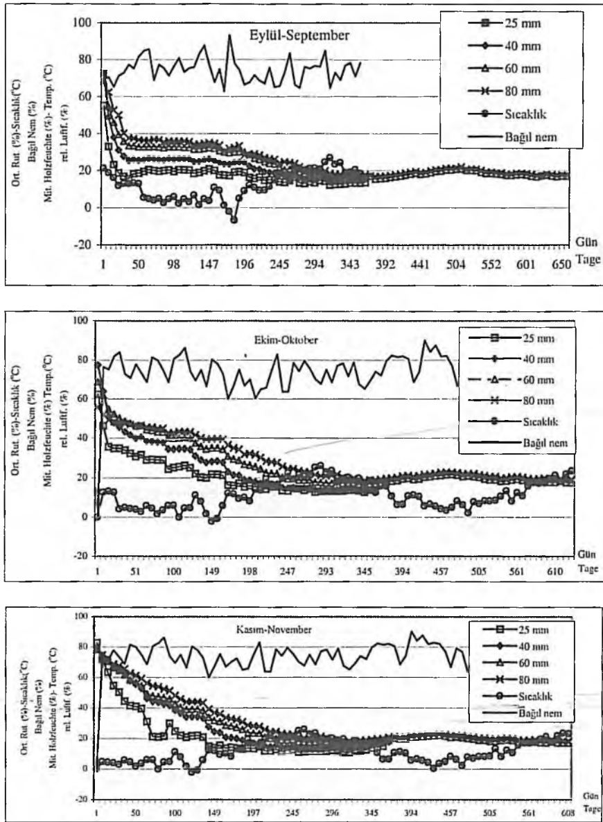
Şekil 2: Eylül, Ekim ve Kasım'86 aylarında başlayan denemelerde elde edilen kurutma eğrileri.
