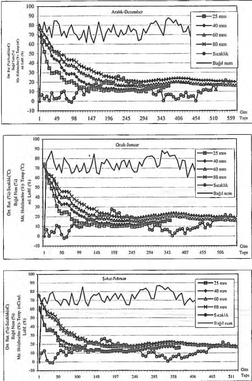
Şekil 3: Aralık'86, Ocak ve Şubat'87 aylarında başlayan denemelerde hüküm süren iklim koşulları ve kurutma eğrileri.
