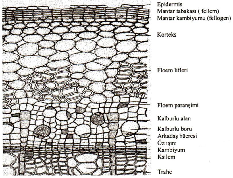
Şekil 2 : Kabukta bulunan önemli hücre ve dokuların şematik görünüşü (WILSON/ LOOMIS 1962).
