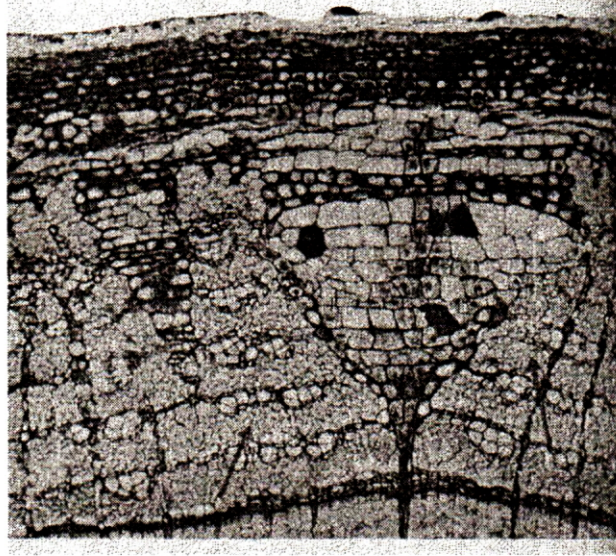
Şekil 3 : Ihlamur gövdesi enine kesitinde kabuğun görünüşü ve floem lifleri (WILSON/ LOOMIS 1962).
