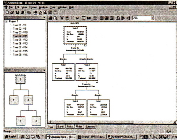
Şekil 7: Gironde orijinin farklı ölçme tarihlere göre analizi.
