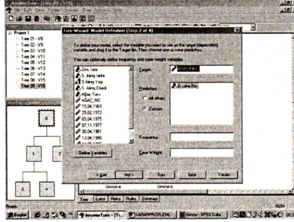
Şekil 5: Değişkenlerin atanması.
