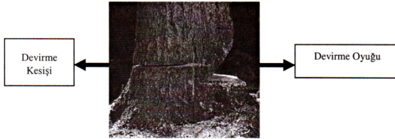
Şekil 2. Devirme oyuğu ve devirme kesişi ( Engür, 2006)
