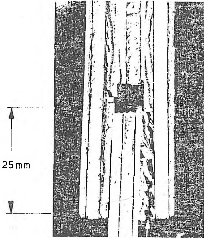
Şekil 3 : Dönme-makaslama kırılması (B.S. 4512'den) Figure 3 : Rolling shear failure (From B.S. 4512)
