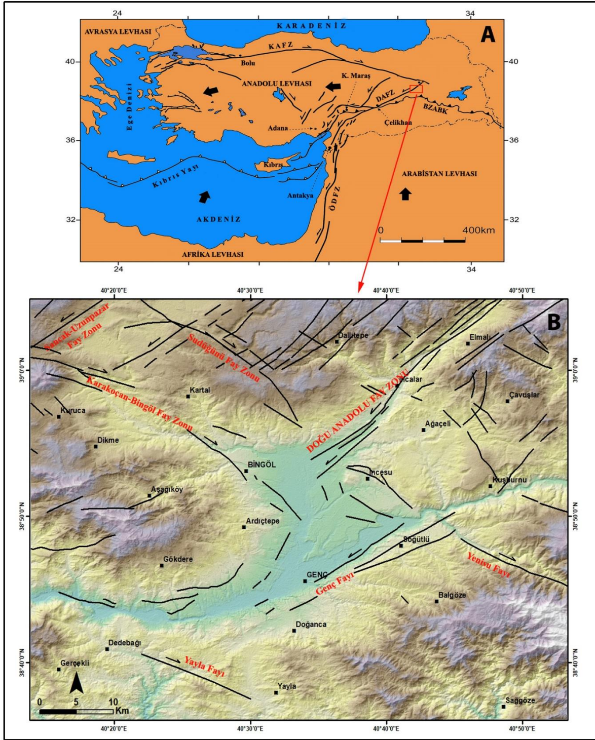
Şekil 1. A) Doğu Akdeniz'in Aktif Tektoniğinin Ana Unsurları. Oklar Levhaların Hareket Yönelerini Göstermektedir BAZBK: Bitlis-Zağros Aktif Bindirme Kuşağı DAFZ: Doğu Anadolu Fay Zonu; KAFZ: Kuzey Anadolu Fay Zonu; ÖDFZ: Ölüdeniz Fay Zonu B) Bingöl Havzası ve Yakın Çevresinin Sayısal Yükselti Modeli ve Havzayı Çevreleyen Aktif Faylar
