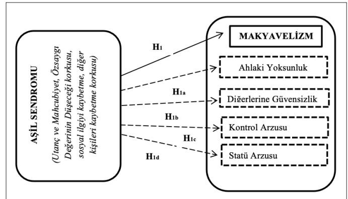
Şekil 1. Araştırma Modeli
