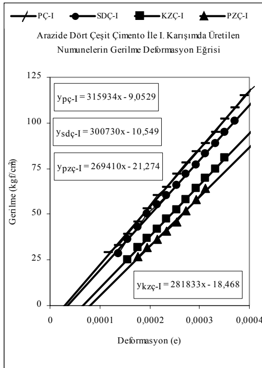
Şekil 9. Araziye Dört Çeşit Çimento İle I. Karışımlarda Üretilen Örneklerin Gerilme Deformasyon Eğrileri.
