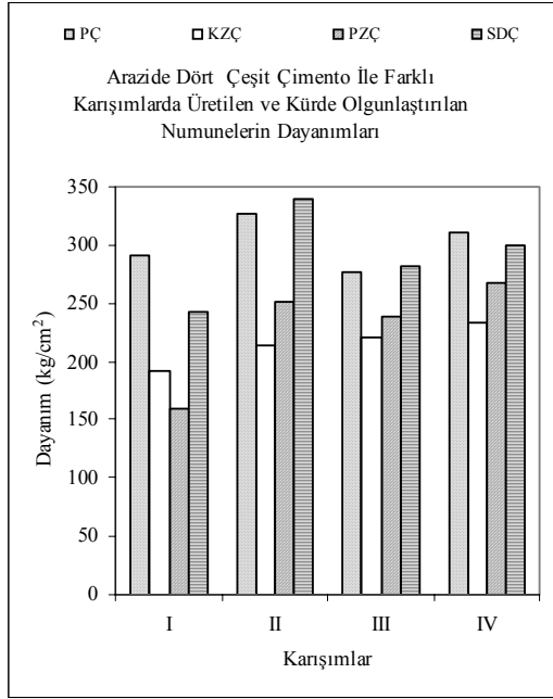
Şekil 8. Araziye Dört Çeşit Çimento İle Farklı Karışımlarda Üretilen ve Kürde Olgunlaştırılan Betonların Ortalama Dayanımları.
