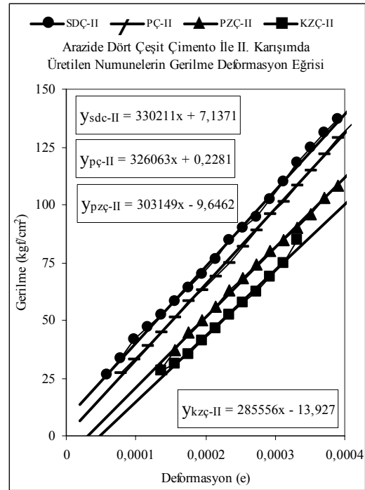
Şekil 10. Araziye Dört Çeşit Çimento İle II. Karışımlarda Üretilen Örneklerin Gerilme Deformasyon Eğrileri.
