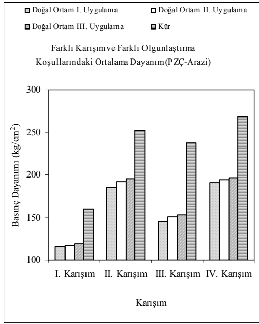
Şekil 3. Arazide Puzolanik Çimentosu İle Dört Değişik Karışım Üretilen Betonların Farklı Olgunlaştırma Koşullarında Ortalama Dayanımları.
