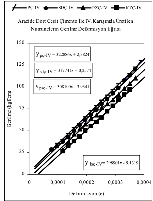
Şekil 12. Arazide Dört Çeşit Çimento İle IV. Karışımlarda Üretilen Örneklerin Gerilme Deformasyon Eğrileri.
