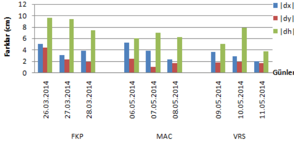
Şekil 7. Ölçü değerleri ile bilinen değerler arasındaki maksimum farklar
