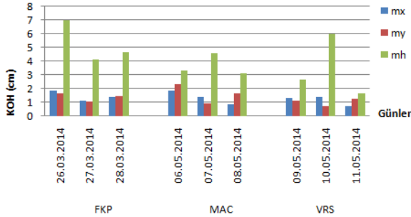
Şekil 8. Düzeltme tekniğine bağlı olarak gerçek değere göre hesaplanan karesel ortalama hatalar
