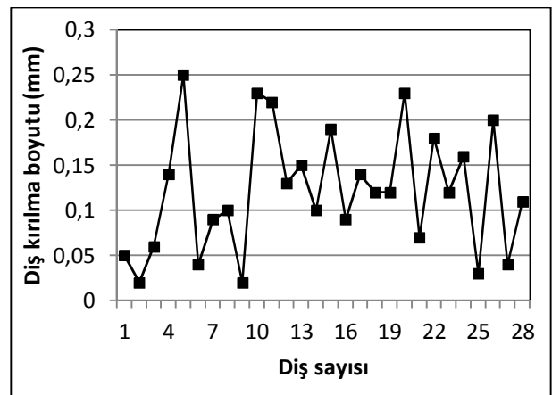
Şekil 7. Diş sayılarına bağlı kırılma boyutları (5. Deney).
