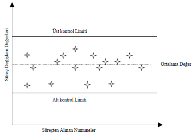
Şekil 2: Örnek süreç kontrol grafiği [12].
