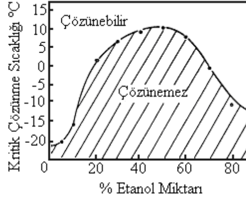
Şekil 1. Etanolün dizel yakıtı içerisinde sıcaklığa göre çözünme yeteneği (Eugene et al., 1984)
