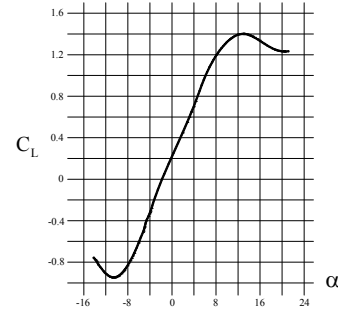
Şekil 4.a. NACA 4415 profili C_L - \alpha eğrisi (NACA 4415 profile C_L - \alpha curve)
