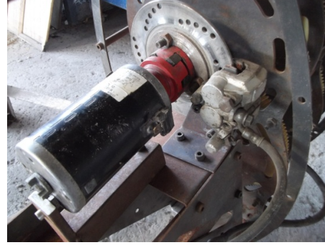
Şekil 9. Kullanılan mekanik fren düzeniği (The mechanical brake assembly)
