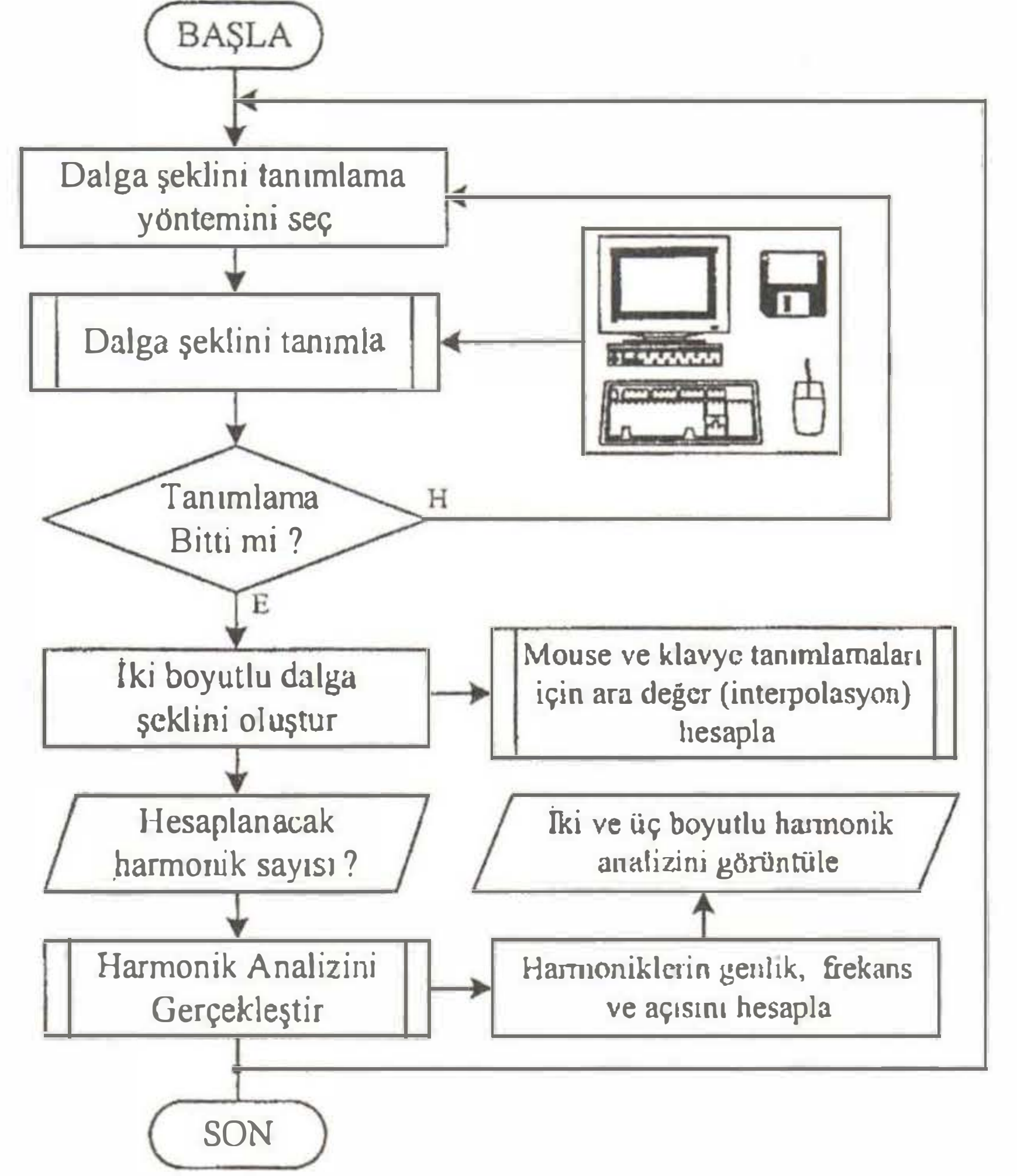
Şekil 1. Program akış diyagramı
