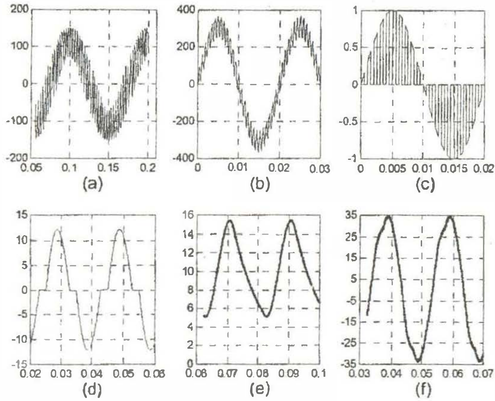
Şekil 4. Harici veriler ile oluşturulmuş dalga şekilleri
