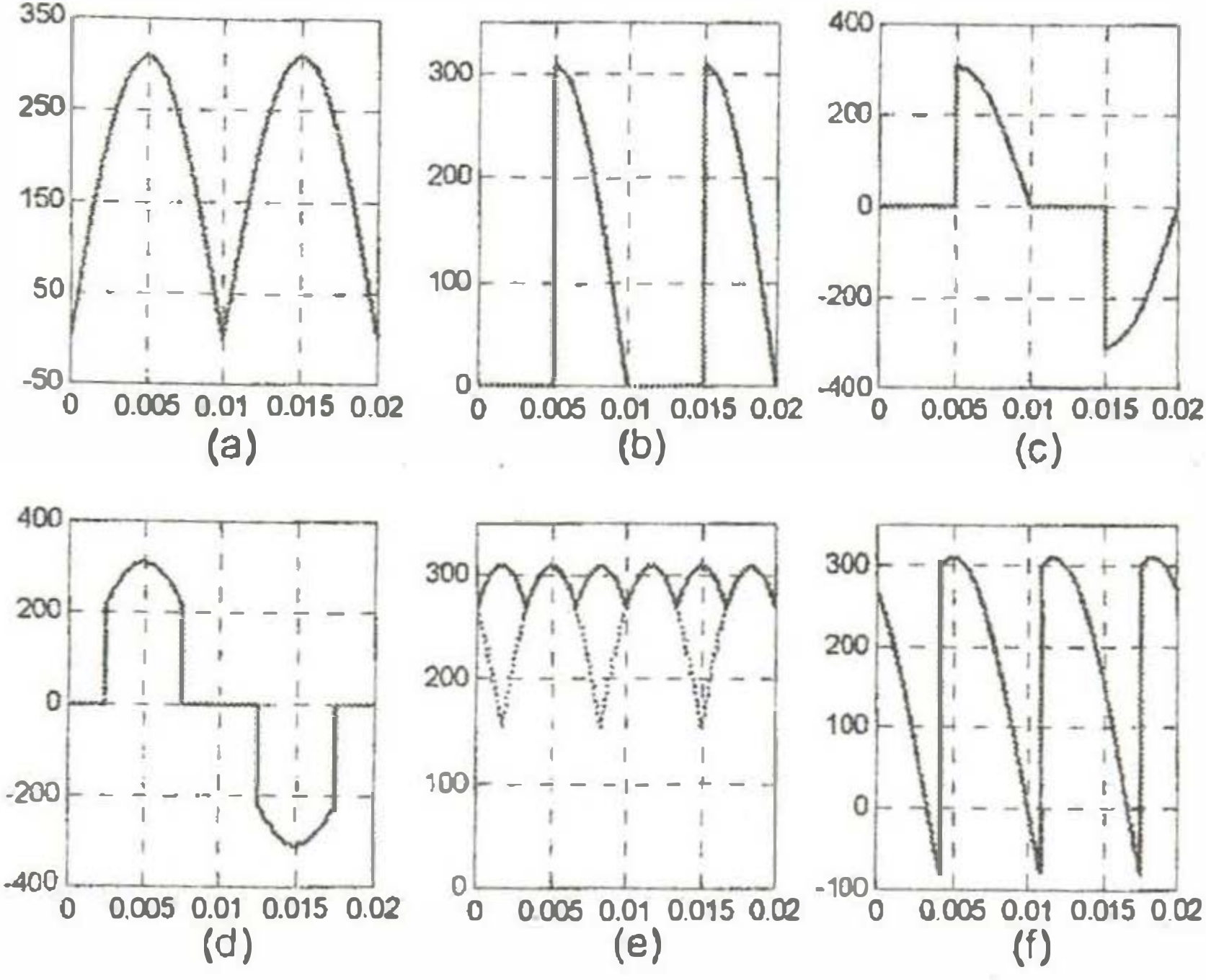
Şekil 3. Parçalı fonksiyonlar ile oluşturulmuş dalga şekilleri
