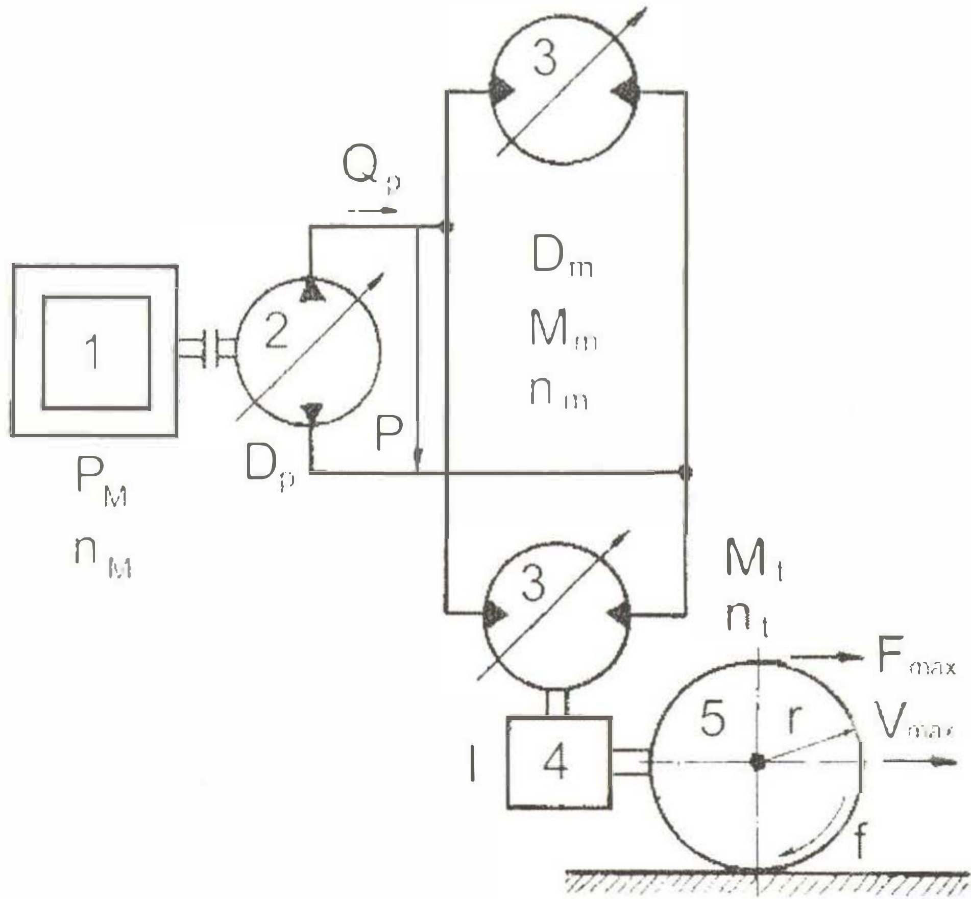
Şekil: 1. Fork-lift için önerilen hidrostatik tahrik tasarım şeması (1: Tahrik motoru, 2: Değişken deplasmanlı aksel pistonlu ana pompa, 3: Hidro-motorlar, 4: Planet dişlili hız düşürücü, 5: Tahrik tekerleği) [5, 7]
