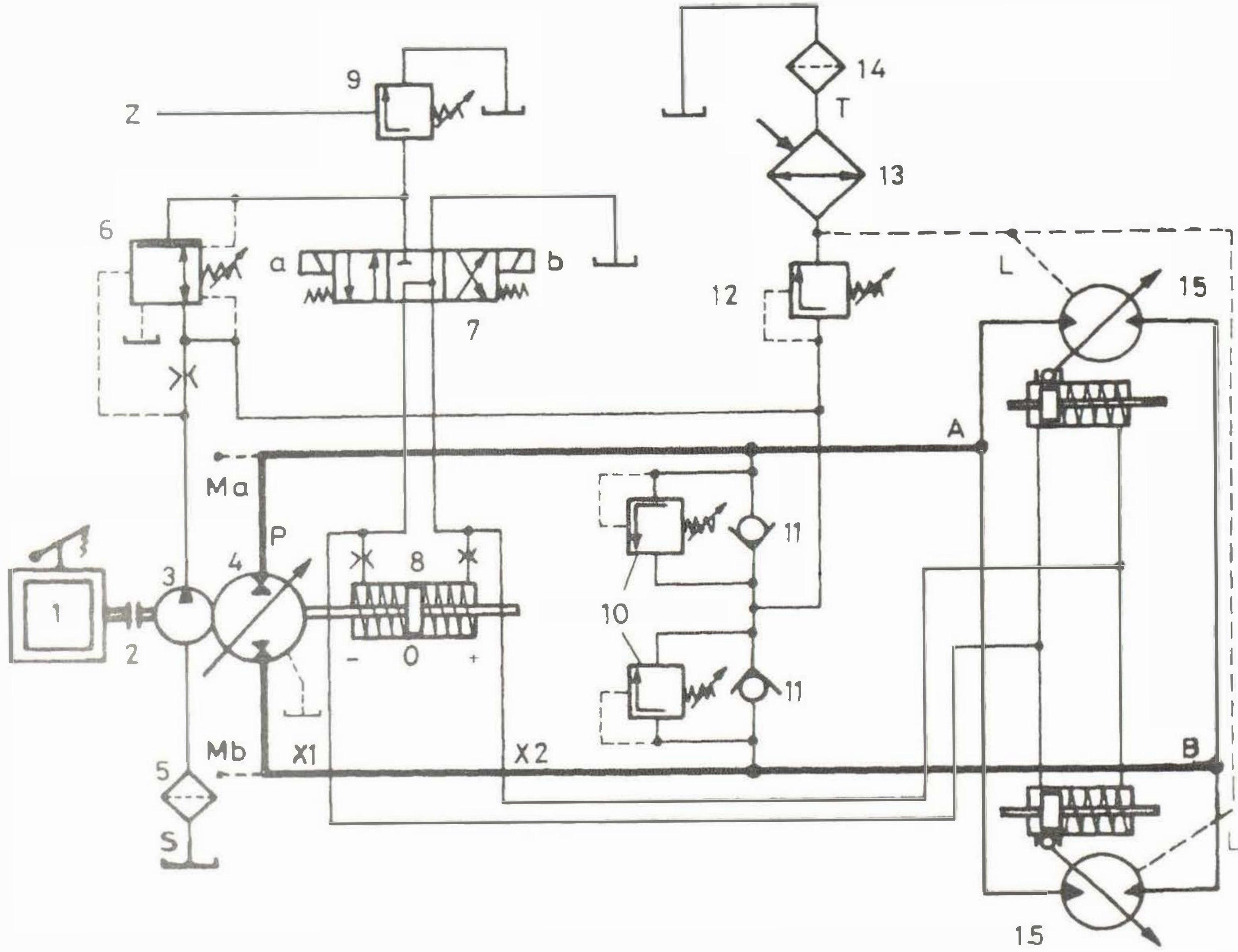
Şekil 4: Hidrostatik tahrik devre şeması (1: Tahrik motoru, 2: Elastik kaplin, 3: Şarj pompası, 4: Değişken deplasmanlı aksel pistonlu ana pompa (A6VM.55.DA), 5: İmiş filtresi, 6: Devire bağımlı hız kontrol valfi, 7: Yön denetim valfi, 8: Pompa deplasmanı ayar organı, 9: Fren valfi, 10: Çapraz valfleri, 11: Besleme çek-valfleri, 12: Basınç denetim valfi, 13: Soğutucu, 14: Dönüş filtresi, 15: Hidro-motorlar (A6VM.55.DA)) [5, 7]
