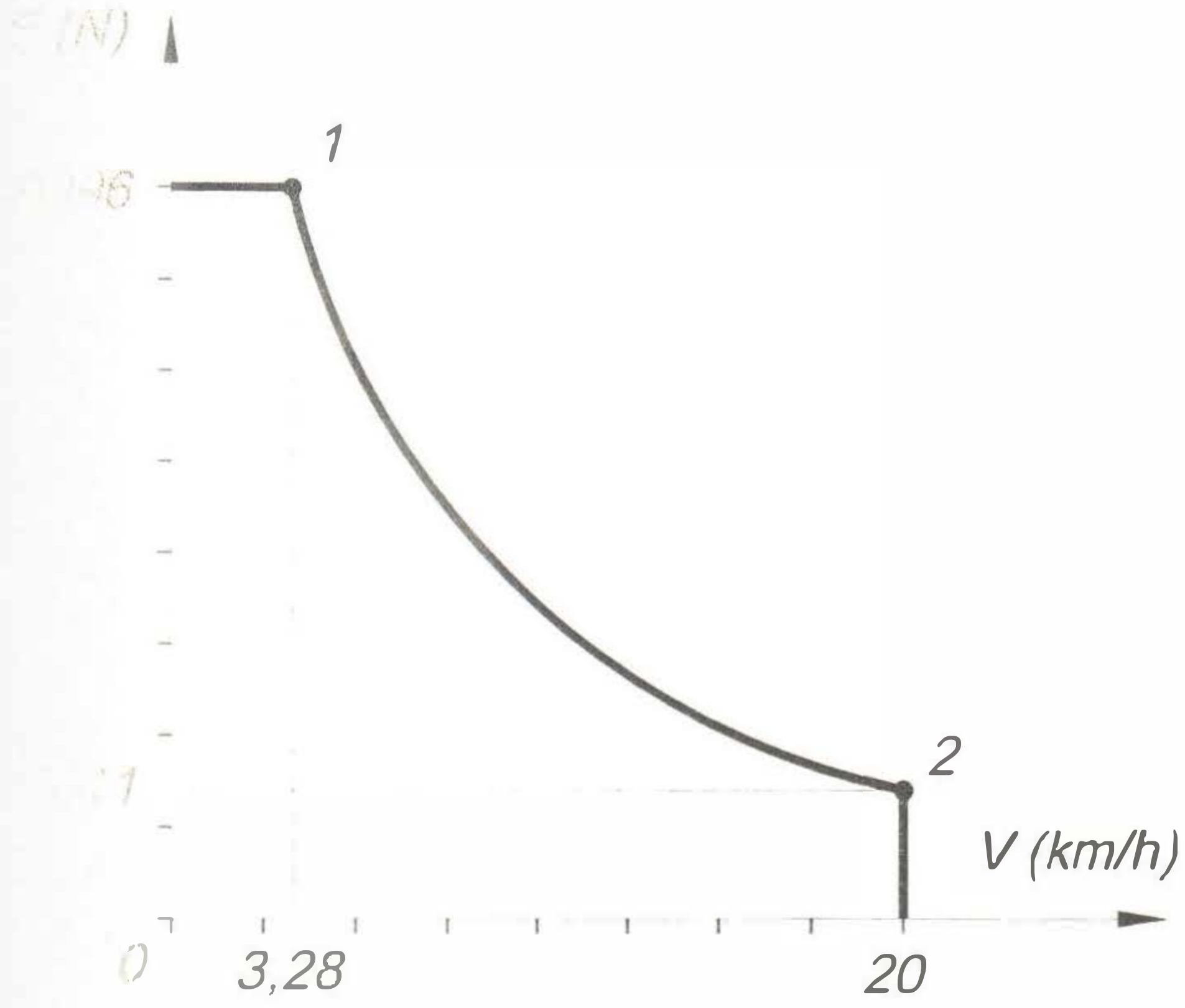
Şekil: 6. Çekiş diyagramı
