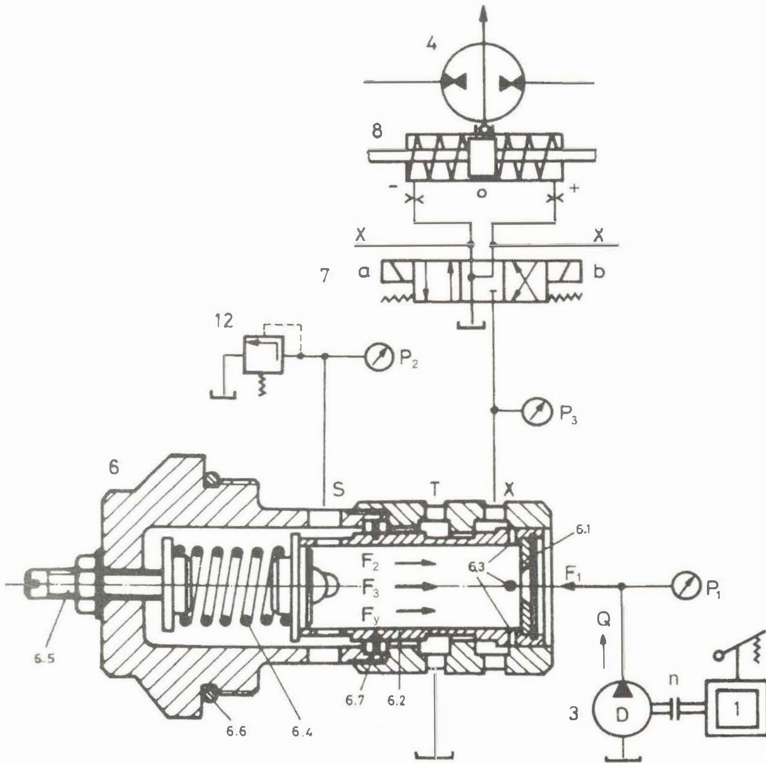
Şekil 4: Devire bağımlı hız kontrol valfi (1: Tahrik motoru, 3: Şarj pompası, 4: Değişken deplasmanlı aksel pistonlu ana pompa, 6: Devire bağımlı hız kontrol valfi, 6.1: Orifis, 6.2: Sürgü, 6.3: Yağ kanalları, 6.4: Ayar yayı, 6.5: Ayar vidası, 6.6: O-ring, 6.7: Tahdit segmanı). [5, 7]
