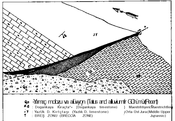
Şekil 7: Manastır D. mekanik dokanağını gösteren şematik profil. Figure 7: The schematic profile showing Manastır D. mechanical contact.
