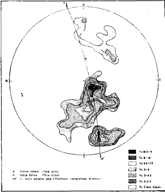
Şekil 10: Kireçlitepe kireçtaşlarında gelişmiş kıvrımların ortalama eksenini ve dalımını gösterir Schmidt diyagramı. Figure 10: Schmidt diagram showing average axis and plunge of folds developed in the Kireçli T. limestone.
