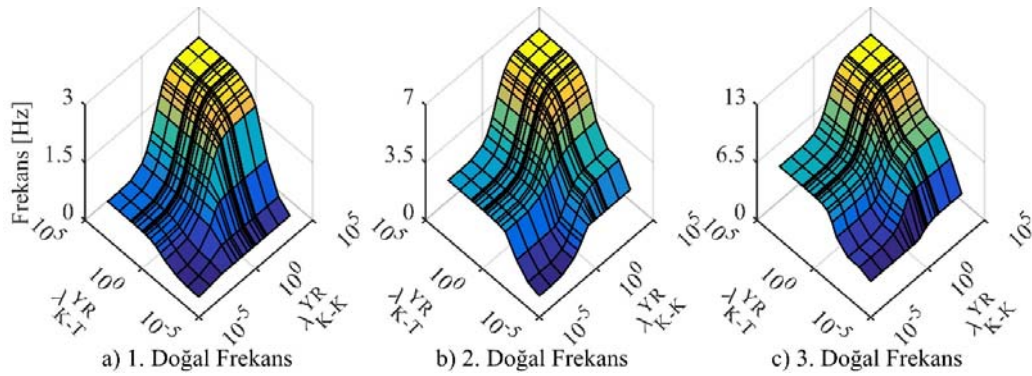
Şekil 16. 6 Katlı 2 Açıklıklı Çelik Çerçevde 1., 2. ve 3. Doğal Frekanslarının Kiriş-Kolon ve Kolon-Taban Bağlantısı Rijitlik Oranları ile Değişimi ( \lambda_{K-T}^{YR} = Kolon-Taban Bağlantı Rijitlik Oranı [ k_{s,kolon}/(EI/L) ];
