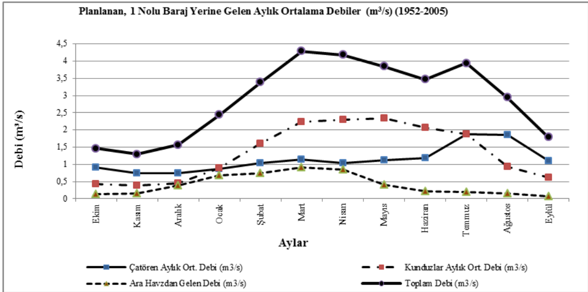
Şekil 13. Baraj gölüne giriş debileri (m³/s)
